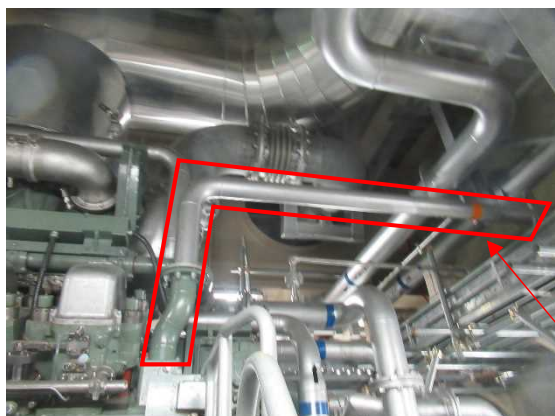
図 1-1 現場状況写真（ディーゼル機関周辺）
