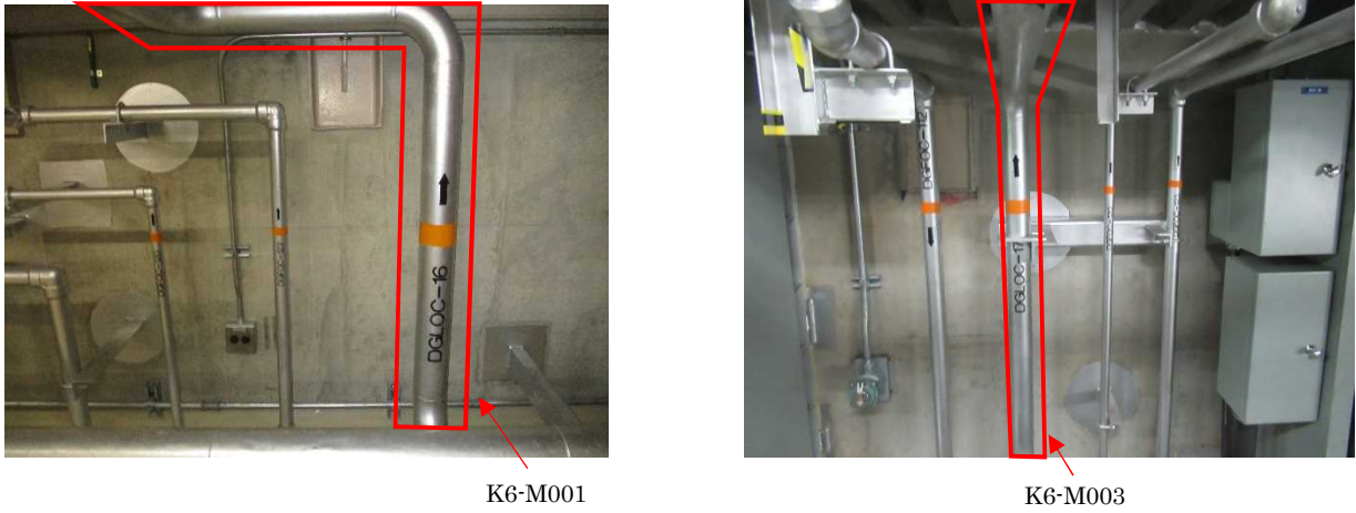
図 1-4 現場状況写真（配管敷設状況）
