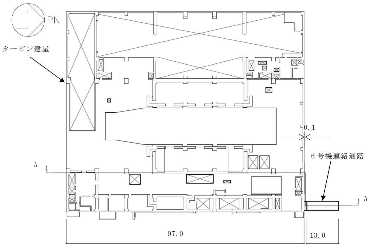
(a) 平面 (T.M.S.L. 20.4m)
