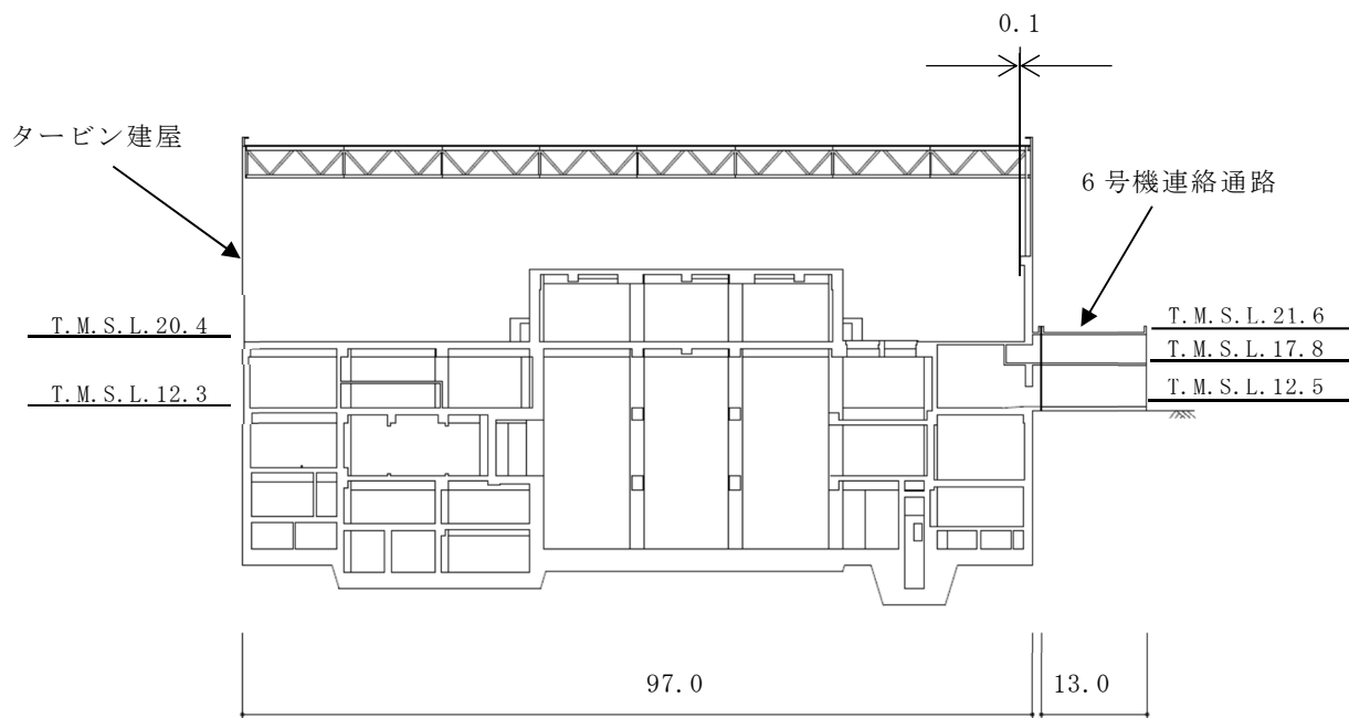
(b) NS 方向断面 (A-A 断面)
