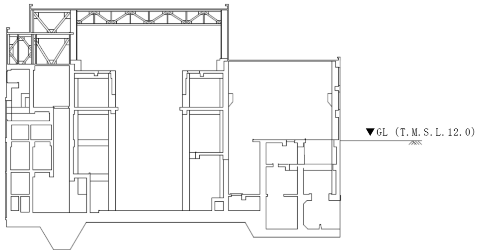
(b) EW 方向断面 (B-B 断面)
