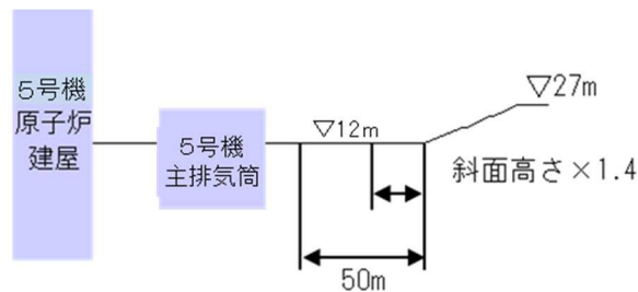
B-B' 断面
