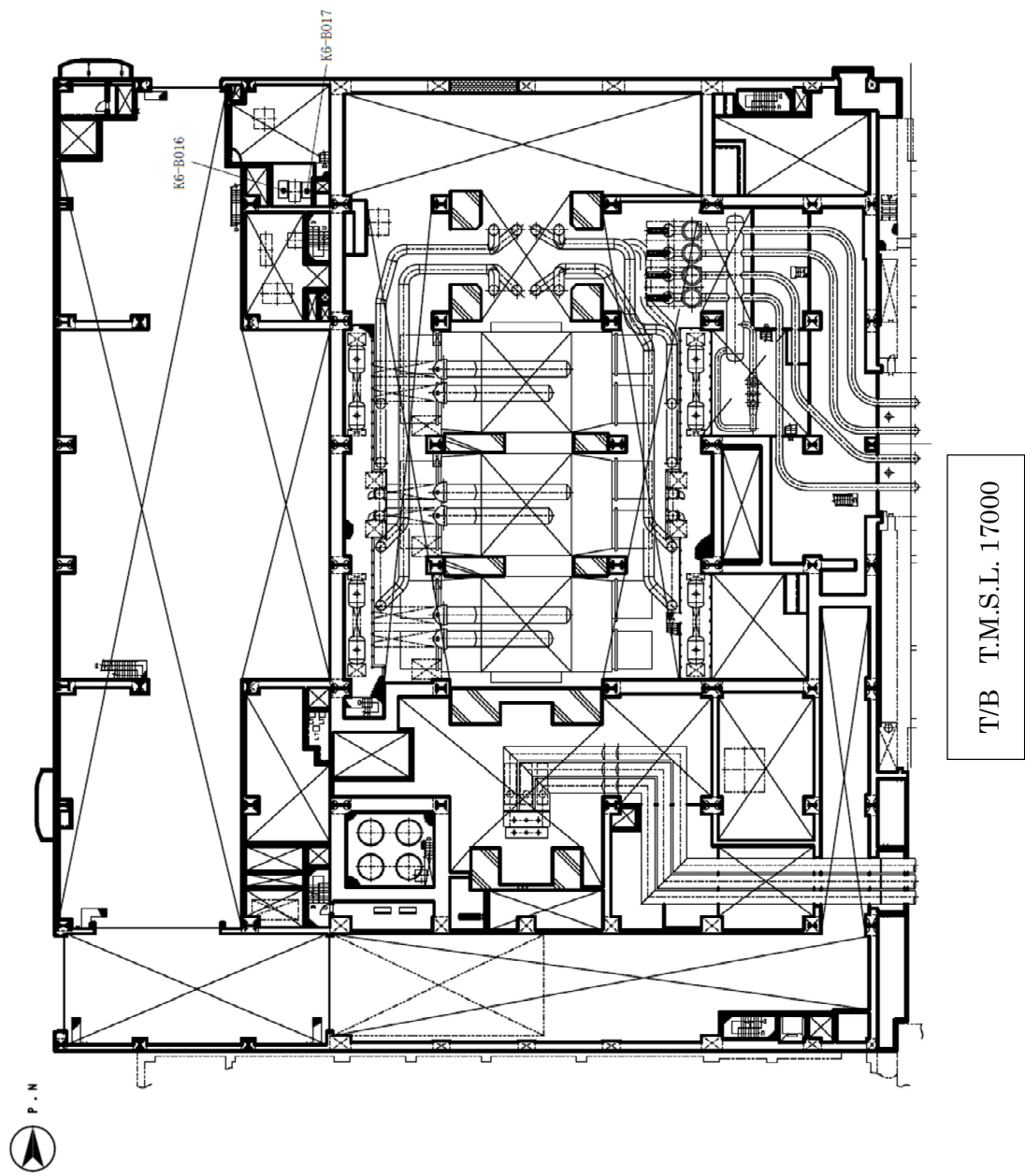
図 6-3-1 柏崎刈羽原子力発電所 6 号機 建屋内上位クラス施設配置図 (28/33)
