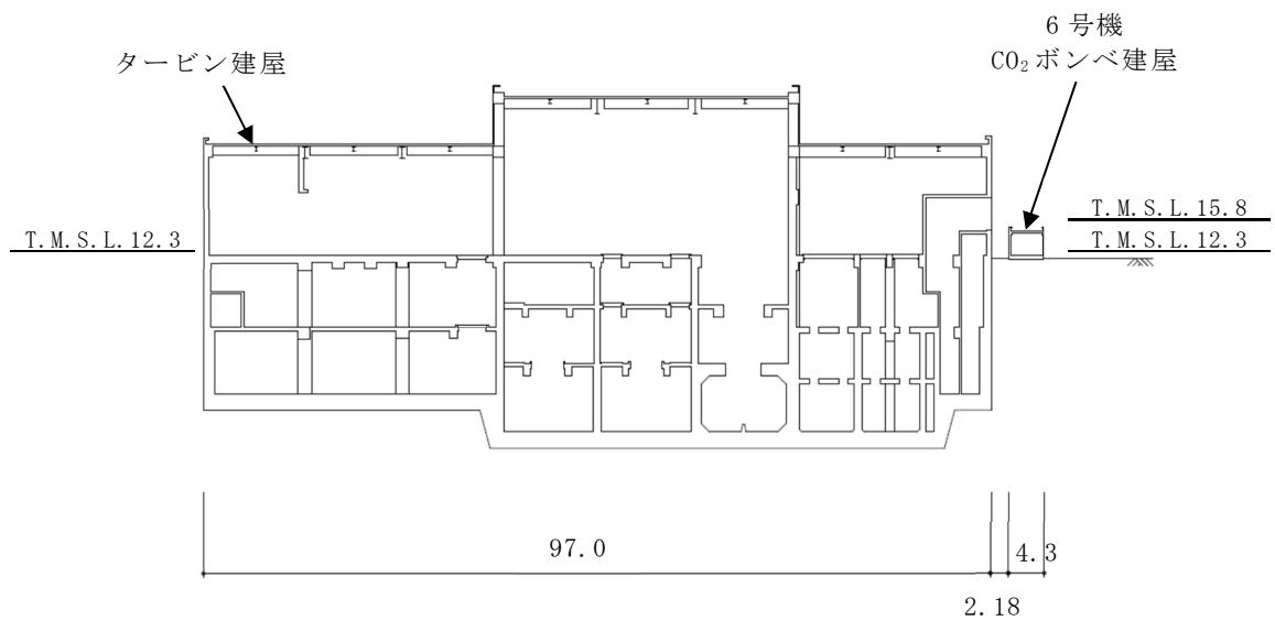
(b) NS 方向断面 (A-A 断面)
