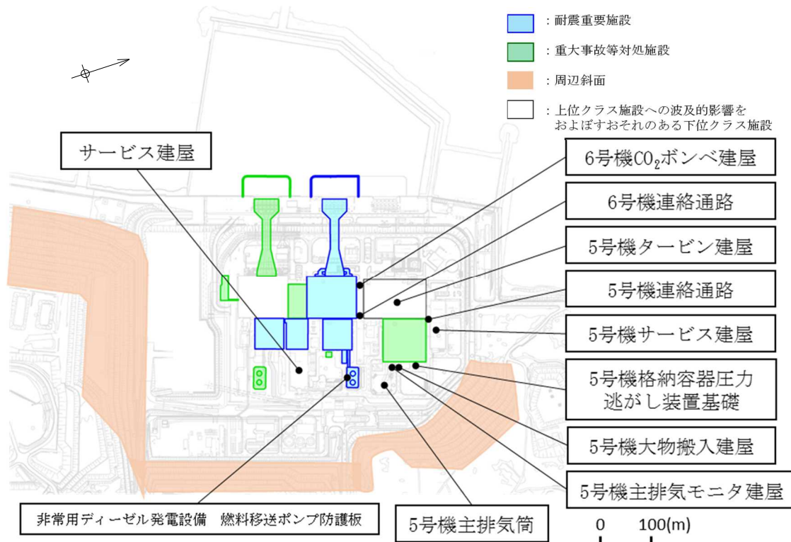
図1 敷地平面図
