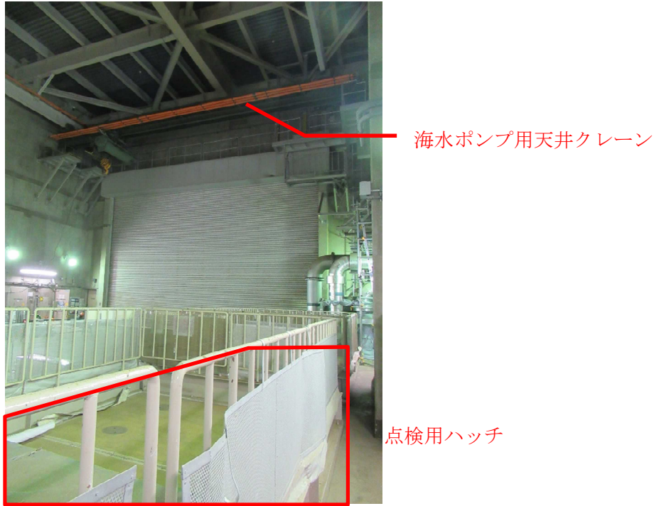
図3 海水ポンプ用天井クレーン設置状況 (6号機北側)
