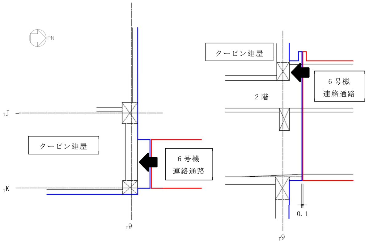
(a) タービン建屋 2 階平面図 (T. M. S. L. 20. 4m)
