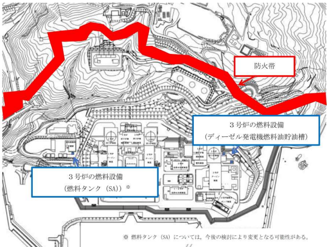
第 41-1-11 図：防火帯と燃料設備（ディーゼル発電機燃料油貯油槽及び燃料タンク（SA））の位置関係
