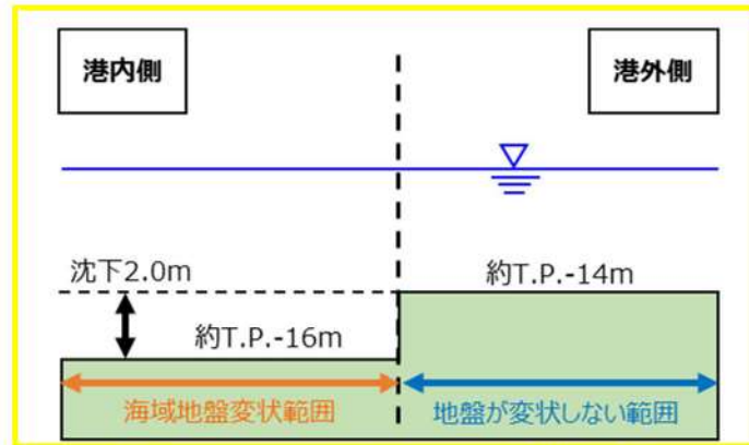
図 2.1.c.c-4 (2) A-A' 断面図
