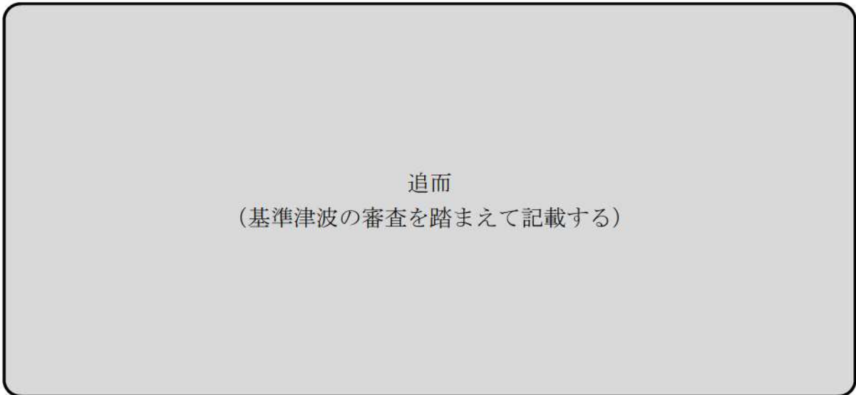
図 2. 1. c. c-6 (55) 敷地（海域）の地盤変状の有無による最大流速分布の比較 (基準津波 ( 追而 ) )
