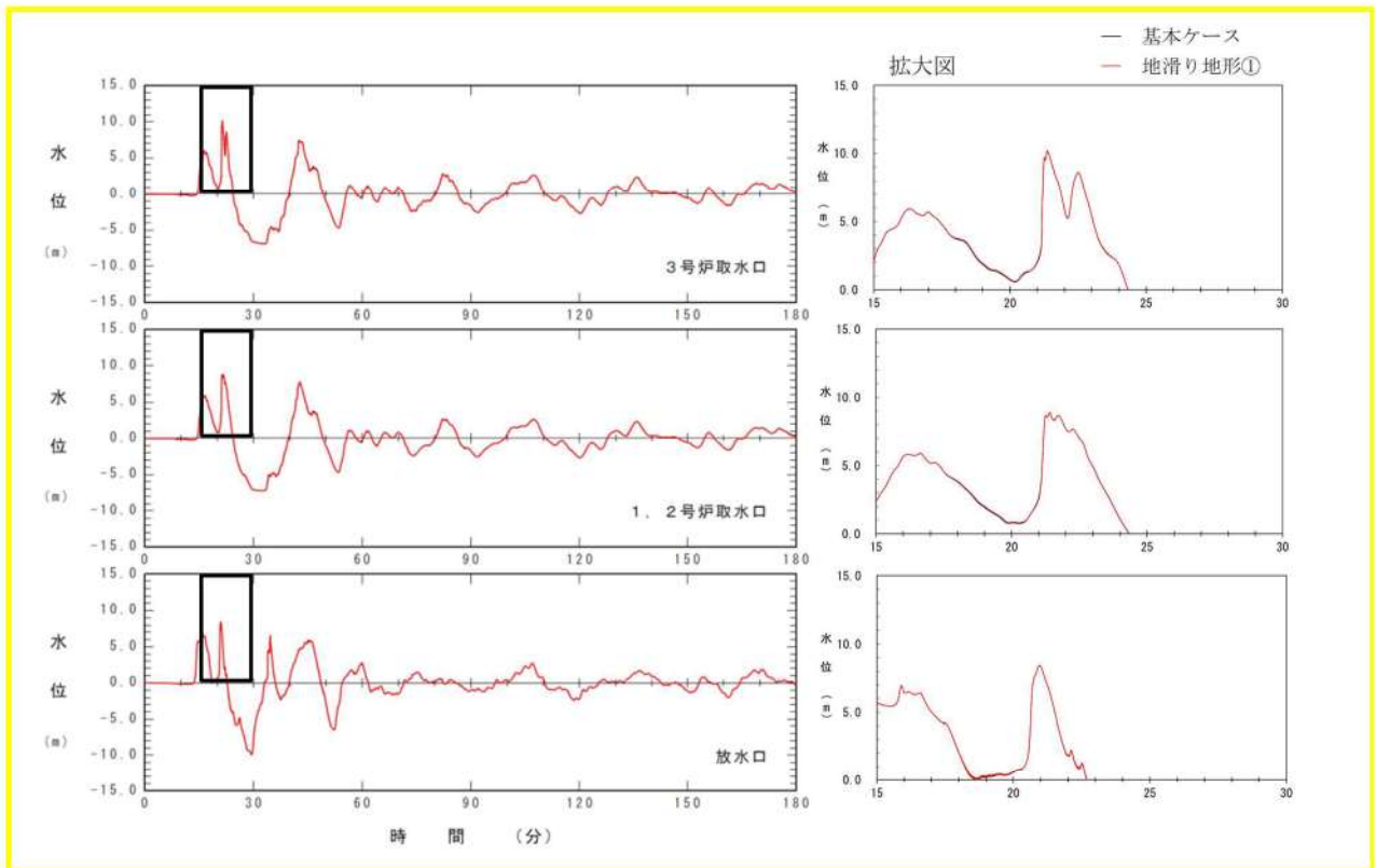
図 2. 1. b. c-1 (4) 地滑り地形①の斜面崩壊の有無による水位時刻歴波形の比較（基準津波（波源 B，防波堤損傷なし））
