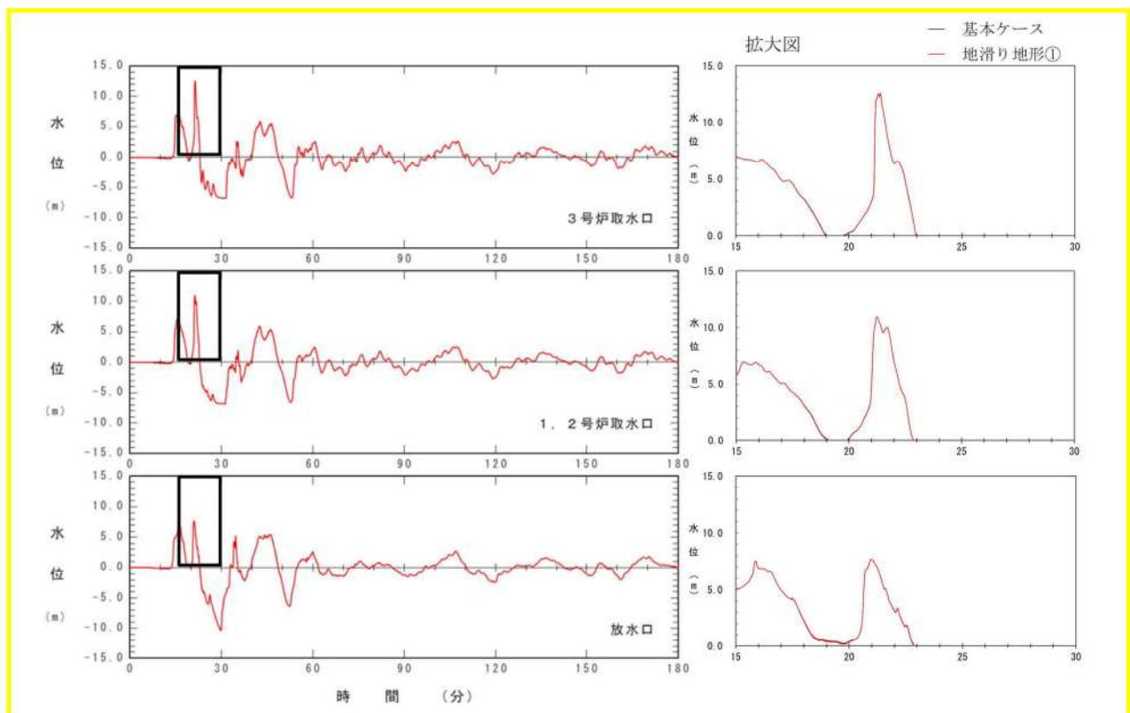
図 2. 1. b. c-1 (6) 地滑り地形①の斜面崩壊の有無による水位時刻歴波形の比較（基準津波（波源B，北防波堤損傷））
