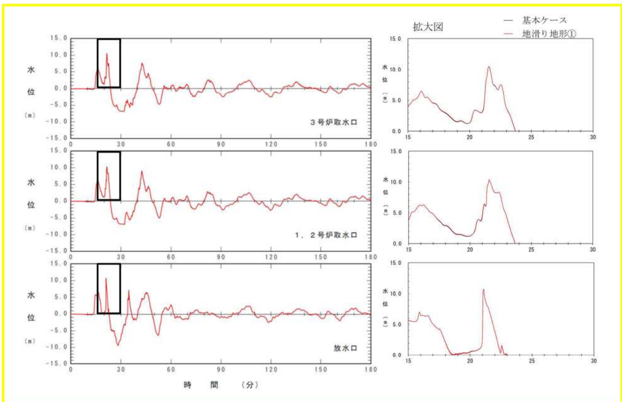
図 2.1.b.c-1 (14) 地滑り地形①の斜面崩壊の有無による水位時刻歴波形の比較（基準津波（波源D，南防波堤損傷））
