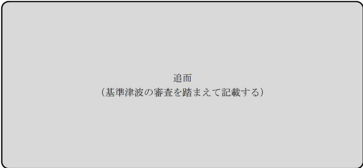
図 2.1.c.c-6 (32) 敷地（海域）の地盤変状の有無による最大水位下降量分布の比較（基準津波（ ））
