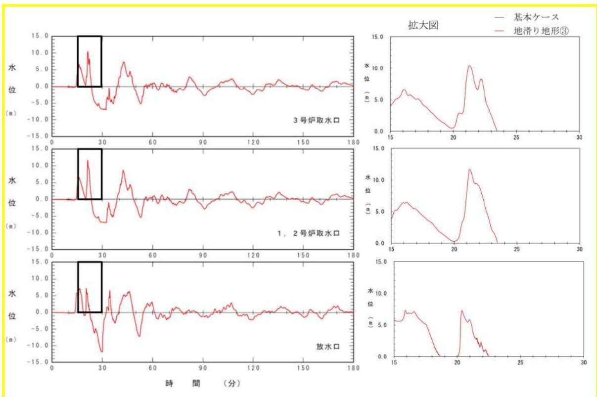
図 2.1. b. c-2 (26) 地滑り地形③の斜面崩壊の有無による水位時刻歴波形の比較（基準津波（波源G，南防波堤損傷））
