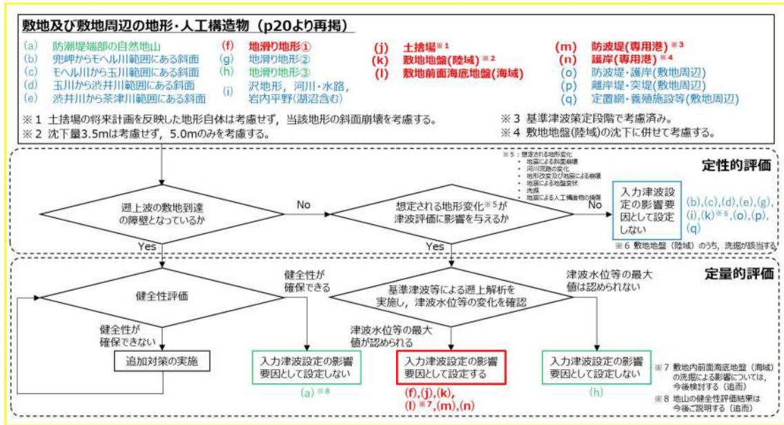
図 2.1. e-1 地震及び津波による地形変化・標高変化の検討結果 (フロー図との関係)
