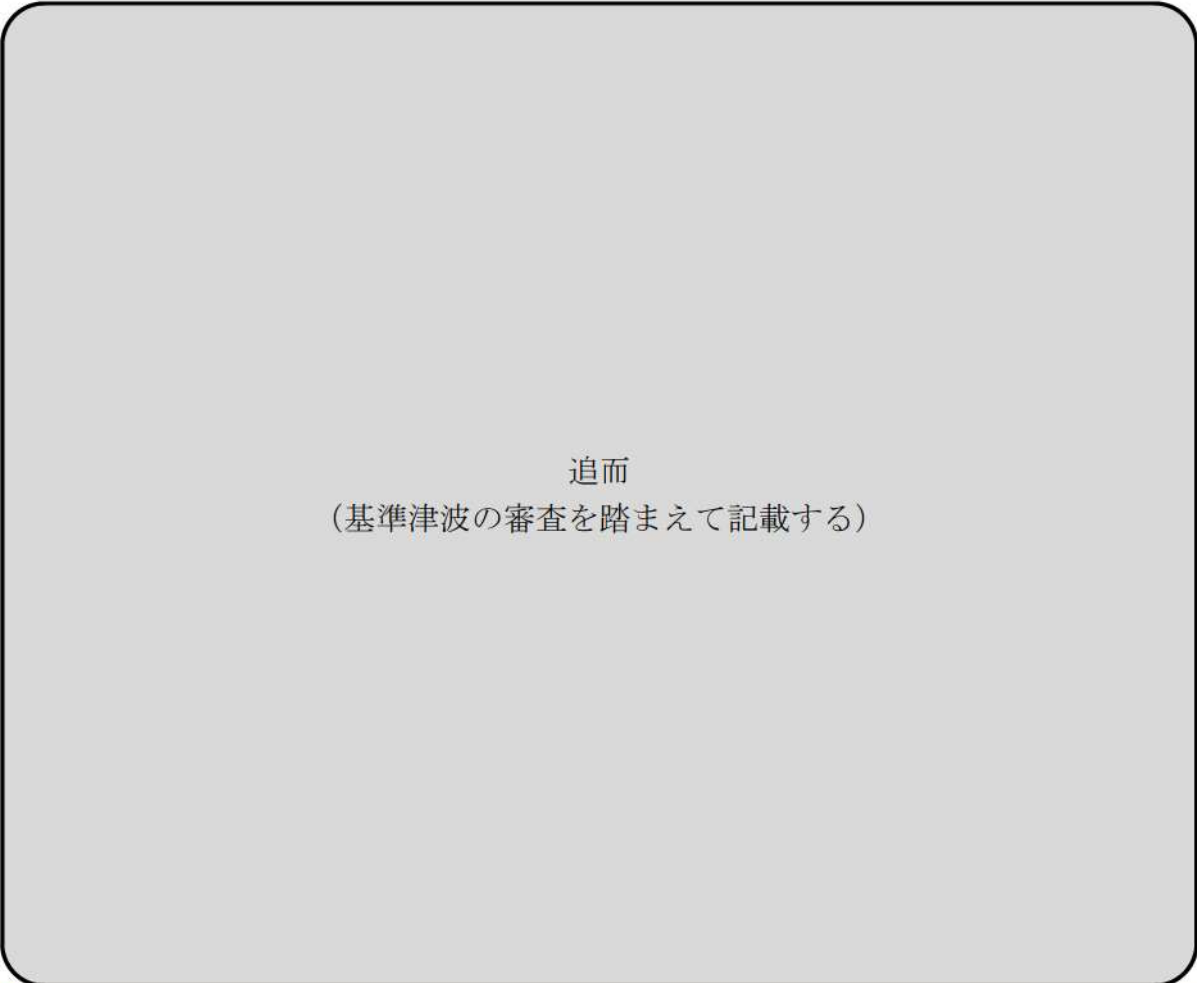
図 2. 1. b. c-1 (40) 地滑り地形①の斜面崩壊の有無による保守性を考慮した時間の比較 (基準津波 追而 )
