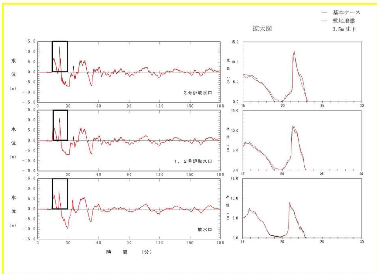
図 2. 1. c. b-22 (28) 敷地（陸域）の地盤変状（3.5m 沈下）の有無による水位時刻歴波形の比較（基準津波（波源H，北防波堤損傷））
