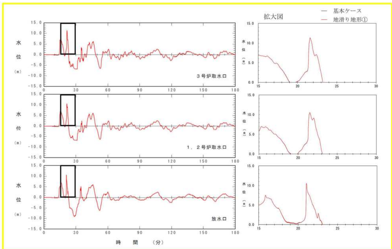
図 2.1. b. c-1 (16) 地滑り地形①の斜面崩壊の有無による水位時刻歴波形の比較（基準津波（波源D，北防波堤損傷））
