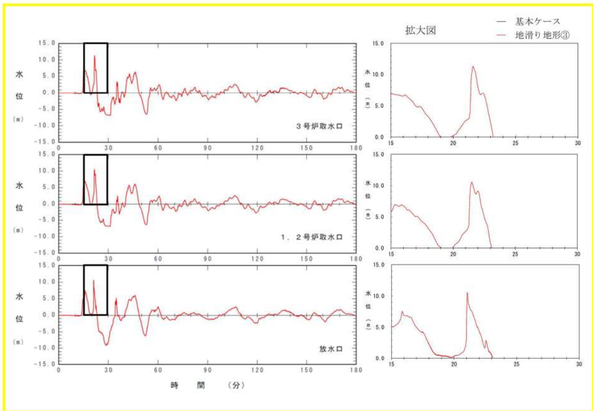
図 2.1.b.c-2 (16) 地滑り地形③の斜面崩壊の有無による水位時刻歴波形の比較（基準津波（波源D，北防波堤損傷））
