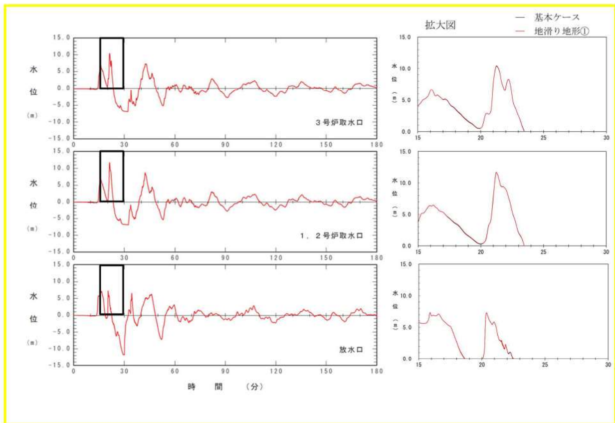
図 2.1. b. c-1 (26) 地滑り地形①の斜面崩壊の有無による水位時刻歴波形の比較（基準津波（波源G，南防波堤損傷））
