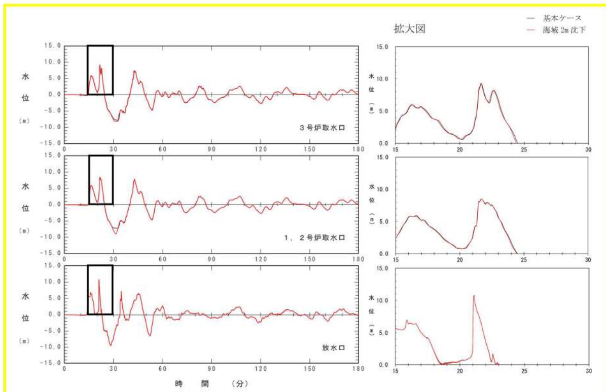
図 2.1.c.c-6 (10) 敷地（海域）の地盤変状の有無による水位時刻歴波形の比較（基準津波（波源D，防波堤損傷なし））
