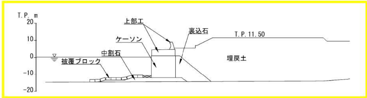
図 2.1.c.b-22 (3) A-A' 断面図
