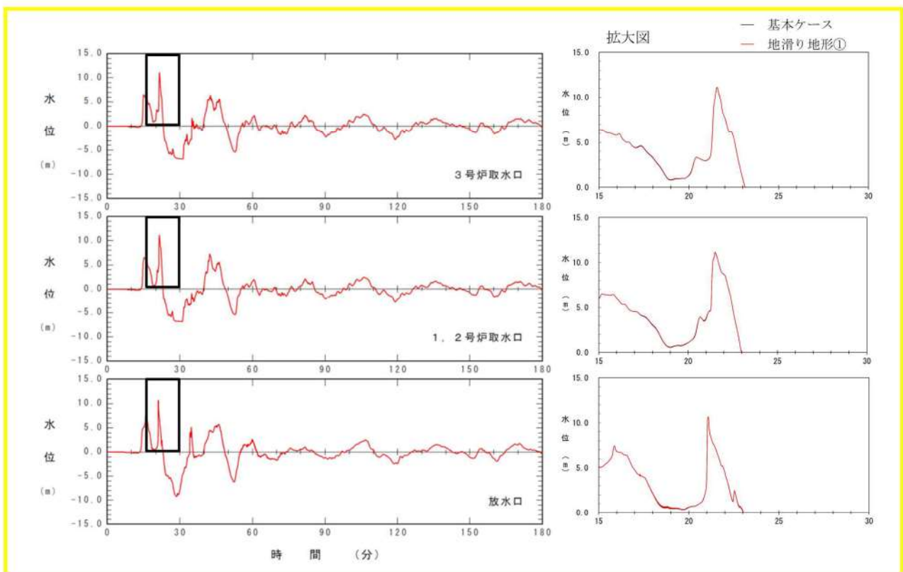
図 2.1.b.c-1 (12) 地滑り地形①の斜面崩壊の有無による水位時刻歴波形の比較 (基準津波 (波源D, 北及び南防波堤損傷))
