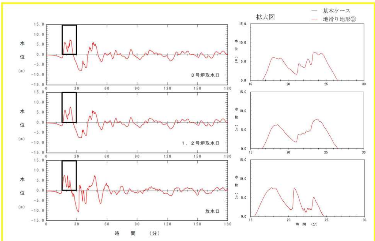
図 2. 1. b. c-2 (2) 地滑り地形③の斜面崩壊の有無による水位時刻歴波形の比較（基準津波（波源A，防波堤損傷なし））
