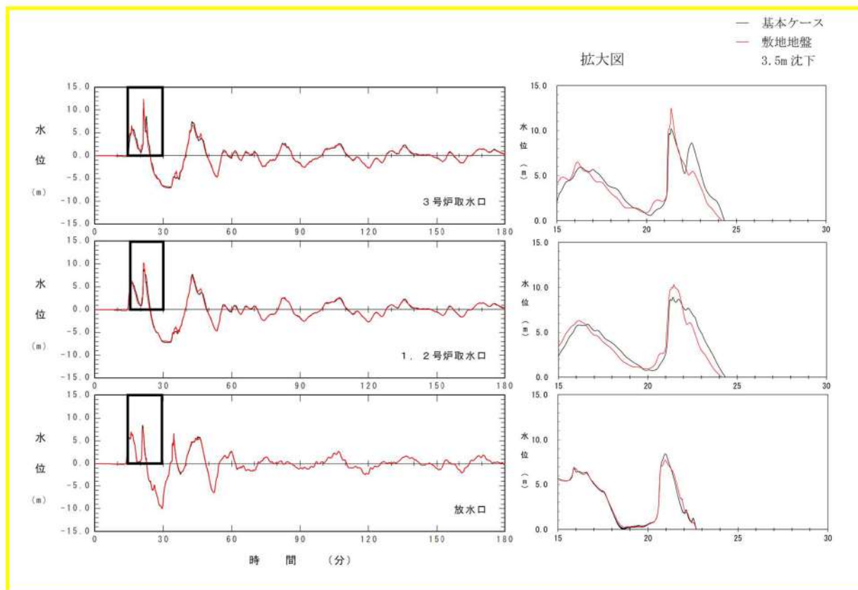
図 2. 1. c. b-22 (4) 敷地（陸域）の地盤変状（3.5m 沈下）の有無による水位時刻歴波形の比較（基準津波（波源B，防波堤損傷なし））
