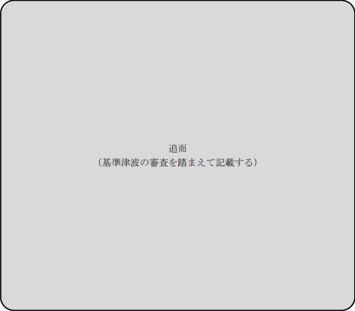
図 2.1.c.c-6 (34) 敷地（海域）の地盤変状の有無による保守性を考慮した時間の比較（基準津波（ 追而 ））
