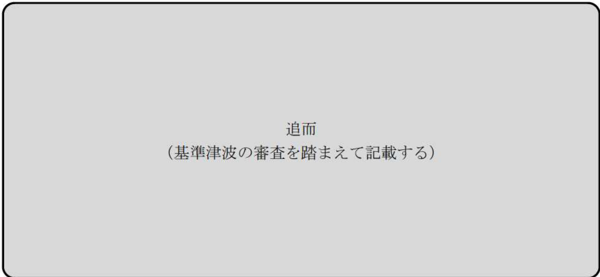
図 2.1.c.b-22 (35) 敷地（陸域）の地盤変状（3.5m 沈下）の有無による最大水位下降量分布の比較（基準津波（ ））
