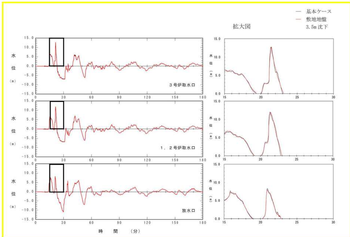
図 2. 1. c. b-22 (18) 敷地（陸域）の地盤変状（3.5m 沈下）の有無による水位時刻歴波形の比較（基準津波（波源E，北及び南防波堤損傷））
