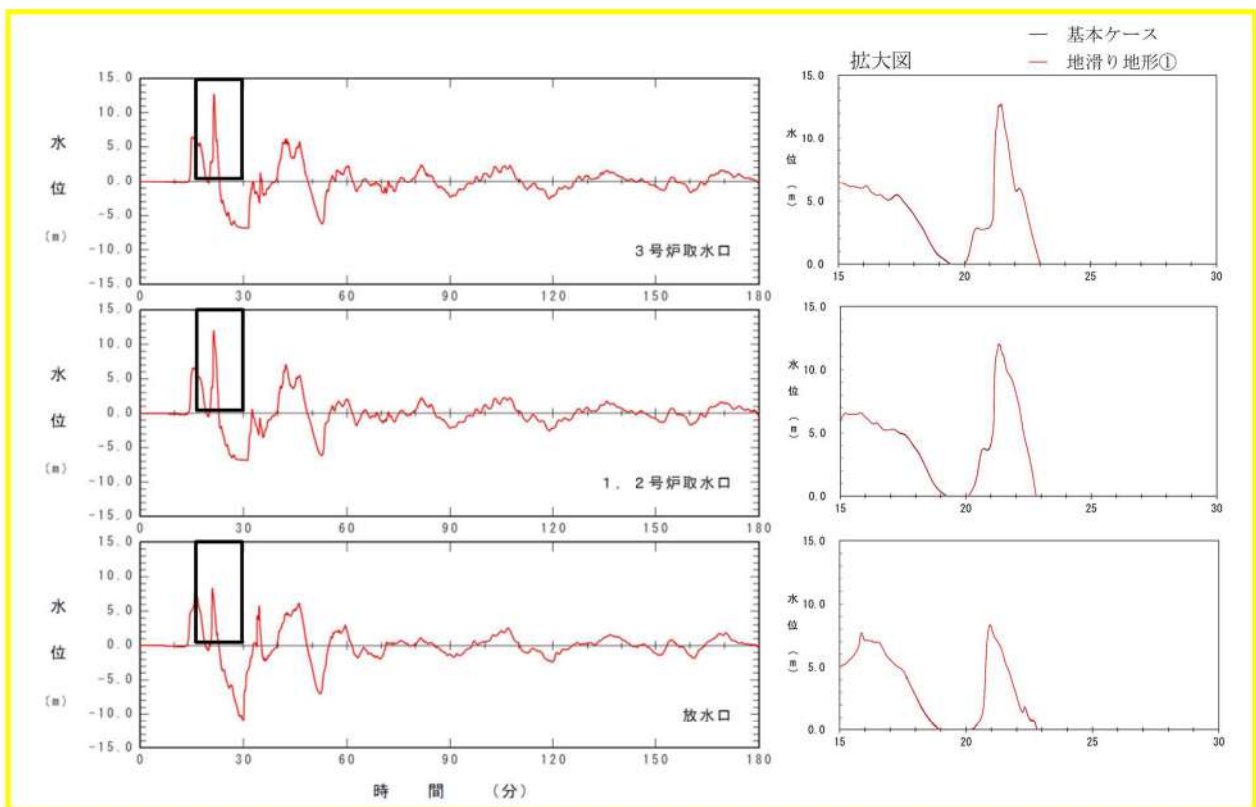
図 2.1.b.c-1 (18) 地滑り地形①の斜面崩壊の有無による水位時刻歴波形の比較 (基準津波 (波源E, 北及び南防波堤損傷))
