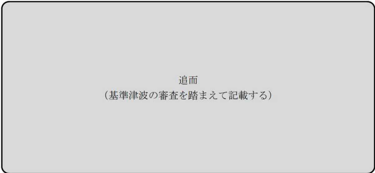
図 2.1.c.c-6 (35) 敷地（海域）の地盤変状の有無による最大水位下降量分布の比較（基準津波（ ））
