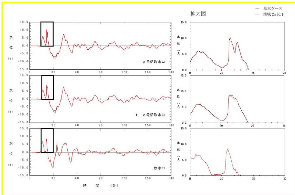
図 2. 1. c. c-6 (4) 敷地（海域）の地盤変状の有無による水位時刻歴波形の比較（基準津波（波源B，防波堤損傷なし））
