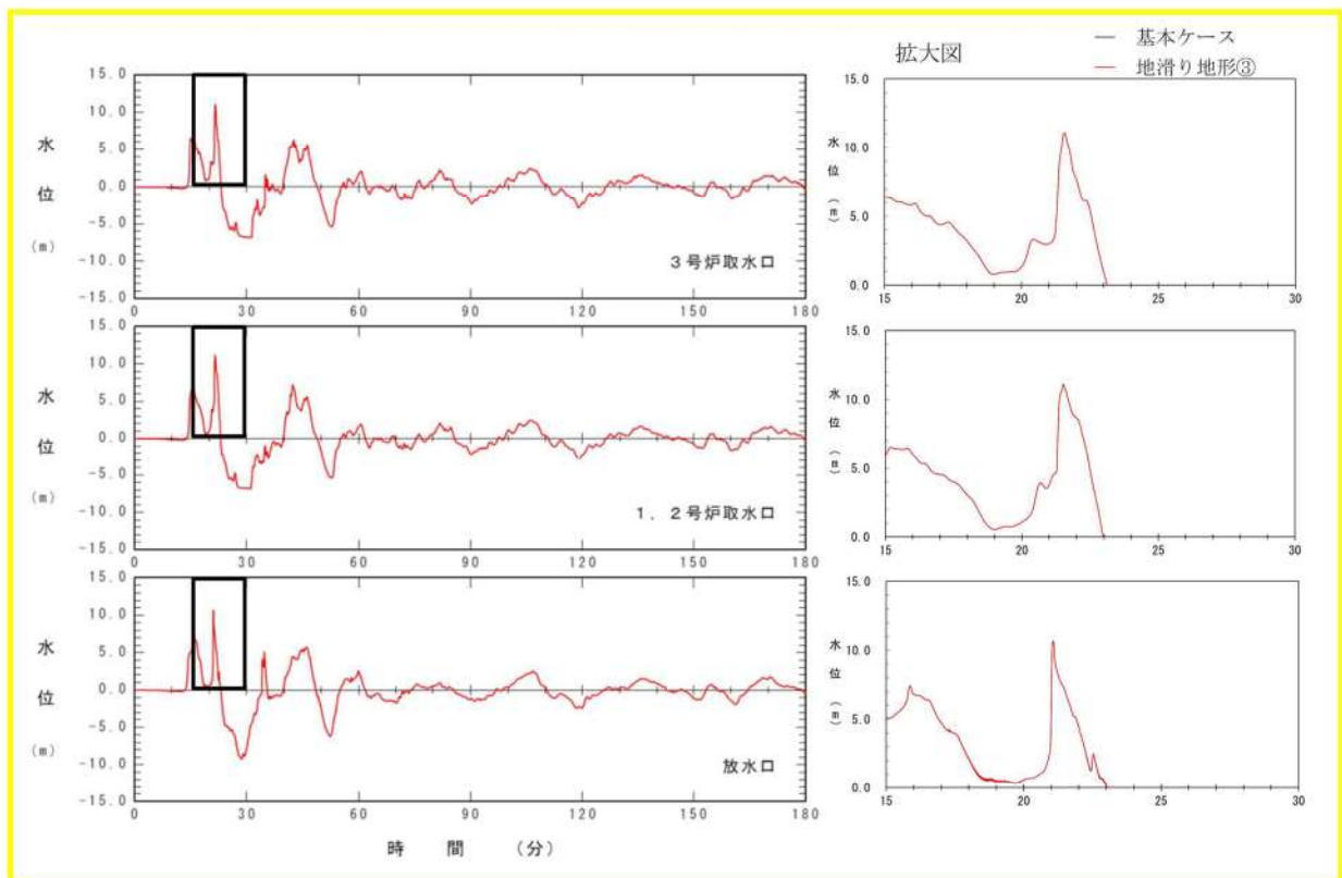
図 2.1. b. c-2 (12) 地滑り地形③の斜面崩壊の有無による水位時刻歴波形の比較（基準津波（波源D，北及び南防波堤損傷））
