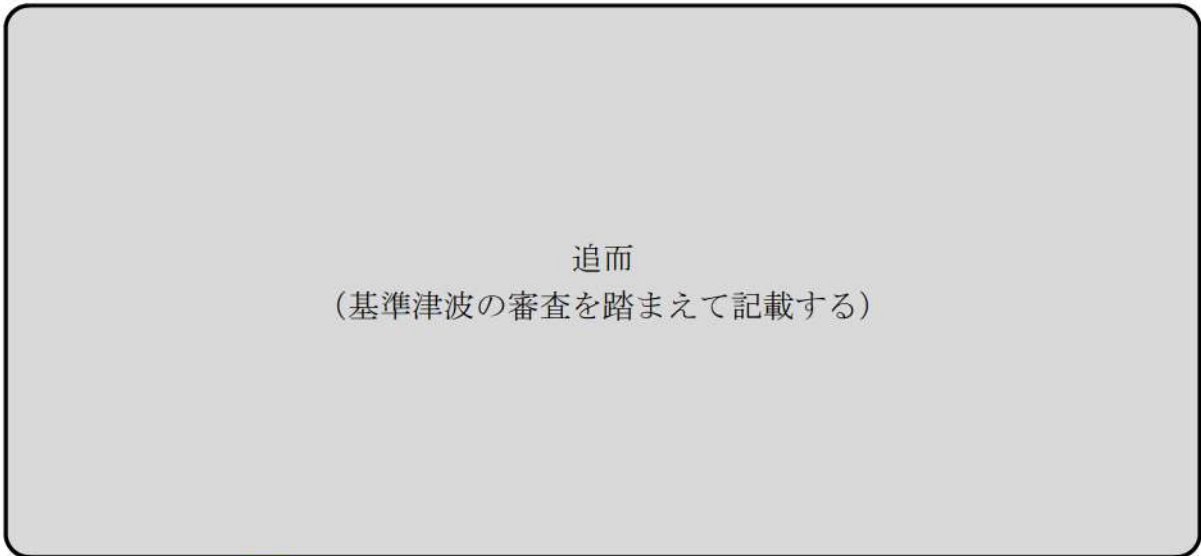
図 2.1.c.b-22 (59) 敷地（陸域）の地盤変状（3.5m 沈下）の有無による最大流速分布の比較（最大流速波源（ ））
