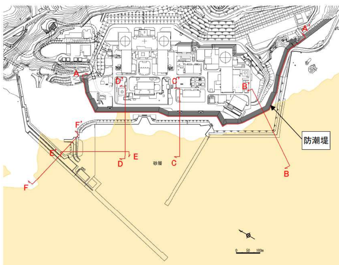
図 2.1.c.b-8 敷地平面図
