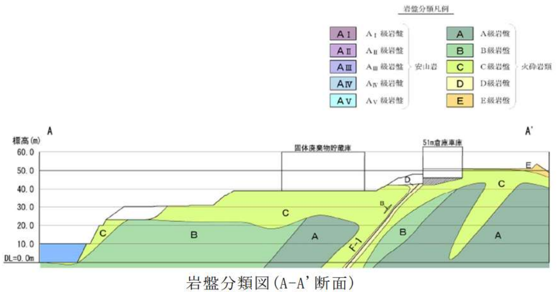
図 2.1. a. c-5 防潮堤（茶津側）地質断面図・岩盤分類図
