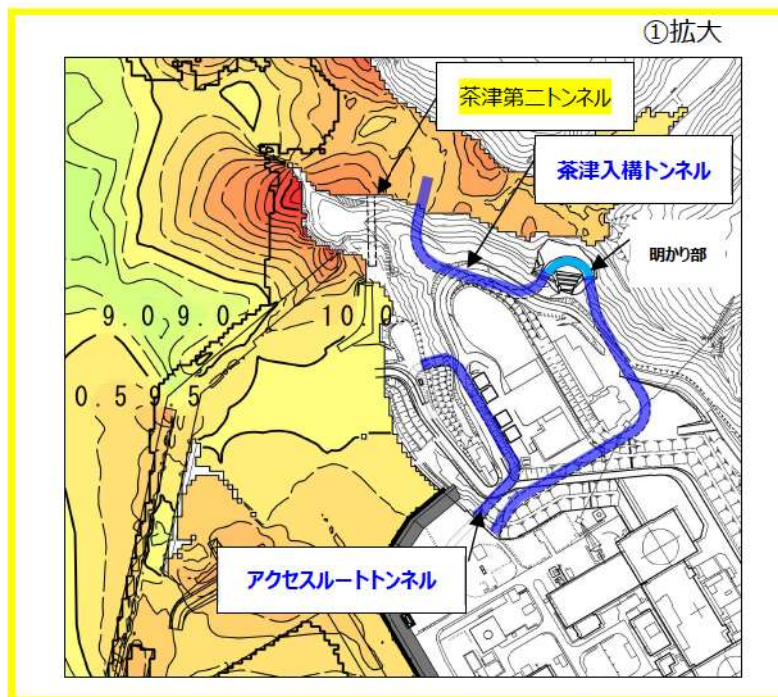
図 1.2.c-1 (2) 最大水位上昇量分布図 (基準津波 (波源D, 北及び南防波堤損傷) ※) ※現時点における最大ケース
