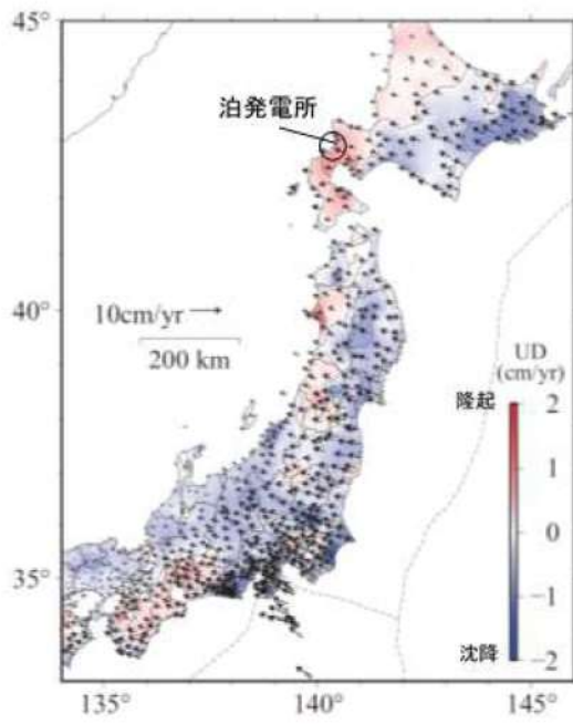
第 1.5-13 図 GEONET による 1997 年 1 月から 2000 年 1 月までの平均変位速度 (Suito, 2018 に加筆)
