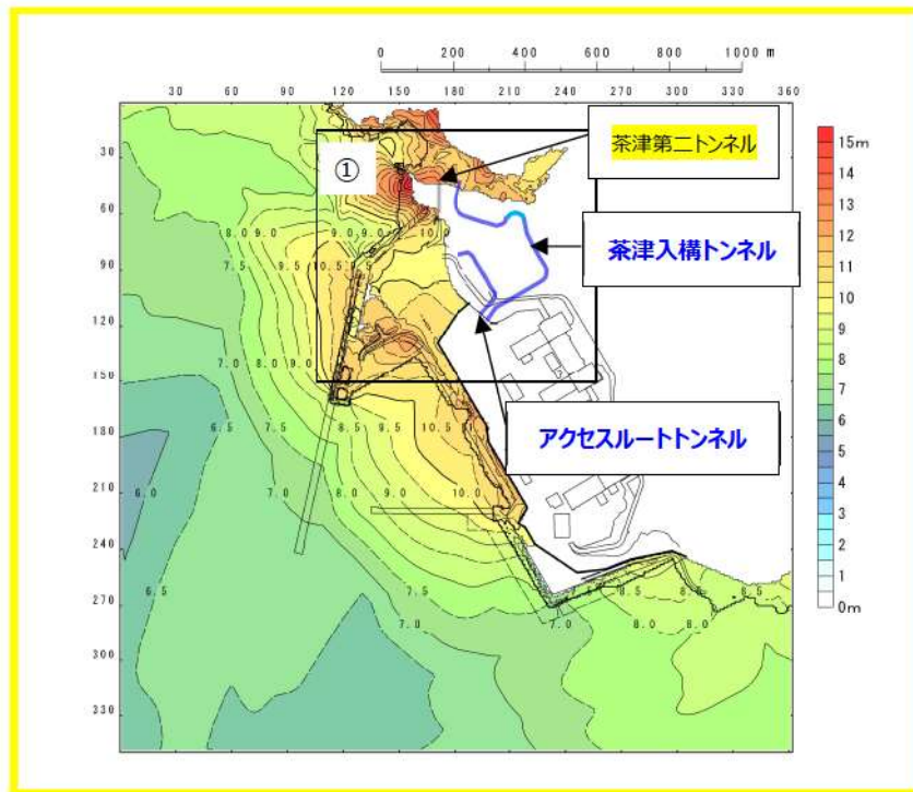
図 1.2.c-1 (1) 最大水位上昇量分布図 (基準津波 (波源D, 北及び南防波堤損傷) ※) ※現時点における最大ケース
