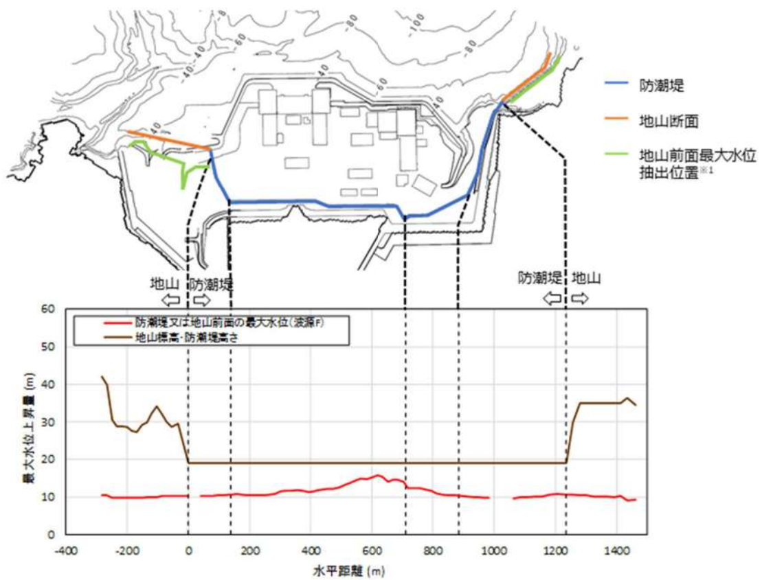
図 1. 2. b-2 防潮堤沿いの最大水位縦断面図 ※2 (基準津波 (波源 F, 北防波堤損傷) ※3 )
