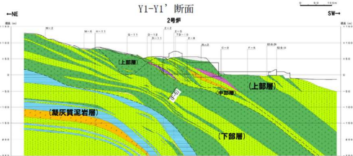
図 2. 1. a. c-2 (2) 泊発電所敷地内地質断面図 (Y1-Y1', Y2-Y2' 断面 令和 3 年 7 月 2 日審査会合資料一部修正)
