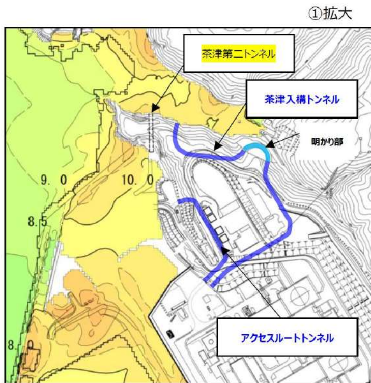
図 1.2.b-1 (2) 最大水位上昇量分布図 (基準津波 (波源 F, 北防波堤損傷) ※) ※現時点における最大ケース
