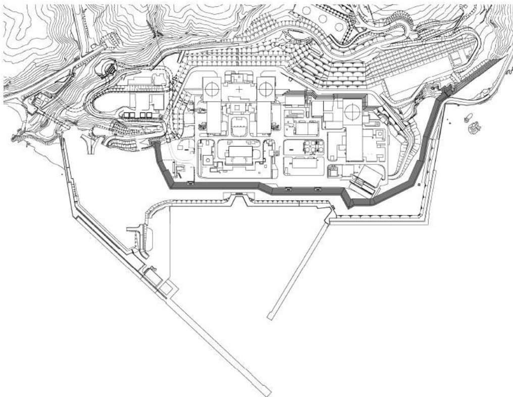
図 1. 1. a. c-4 敷地平面図
