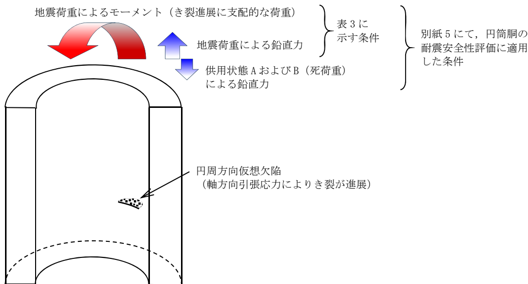
図 1 原子炉圧力容器円筒胴の中性子照射脆化を考慮した評価条件の内訳
