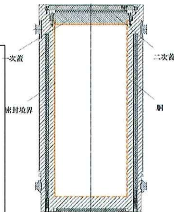
閉じ込め構造図
