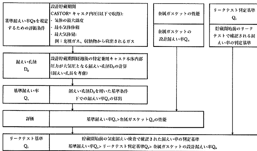
閉じ込め機能評価フロー
