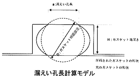
漏えい孔長計算モデル
