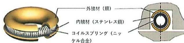
金属ガスケット構造
