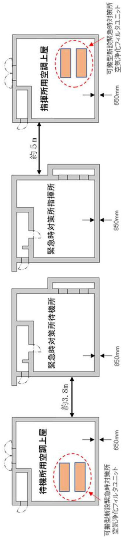
図2.4-23 可搬型緊急時対策所空気浄化ファン及びフィルターユニット設置位置
