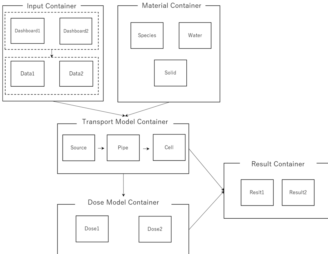
図1 GoldSimにおける全体的なモデルコンテナの枠組み
