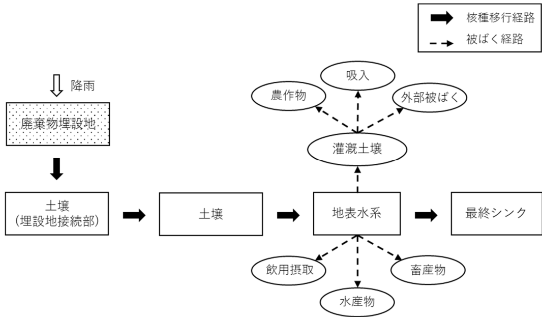
図3 トレンチ処分評価モデル概念図
