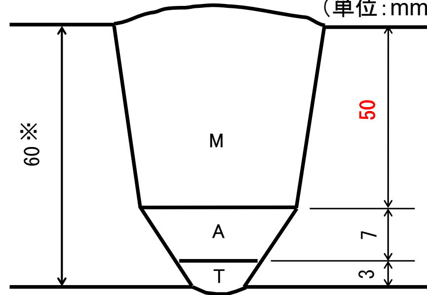
許容される実機溶接の例
