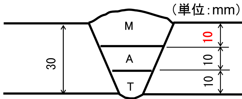
認証試験の溶接厚さ
