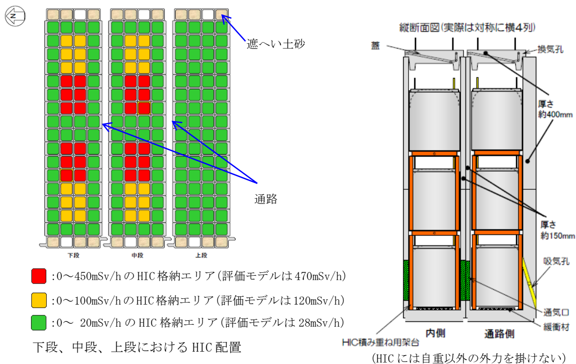
図10 ボックスカルバート概要図
