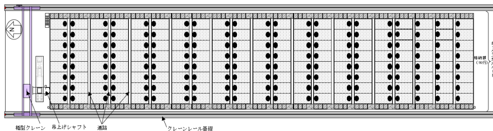
図 7 漏えい検出器設置図
