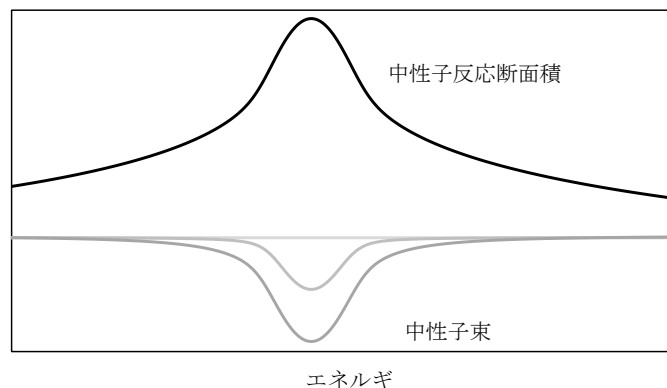
図 中性子反応断面積と中性子束
