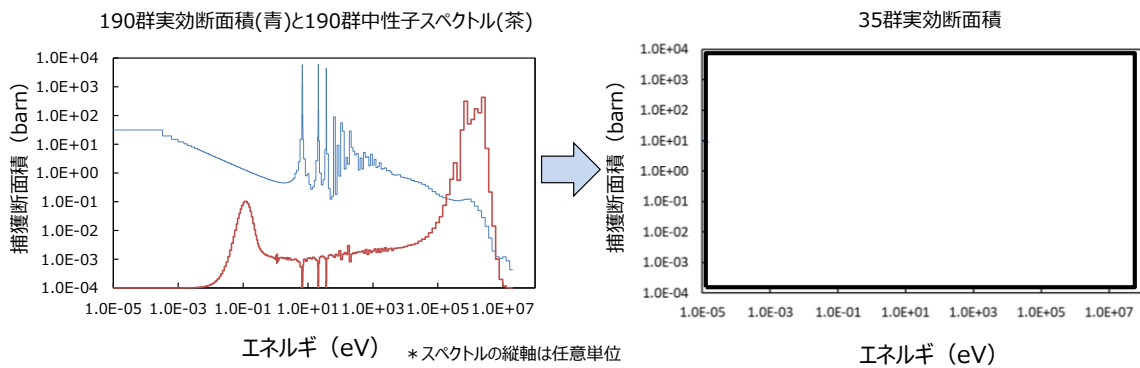
図 1.4-4 中間エネルギー群（35 群）実効断面積の計算
