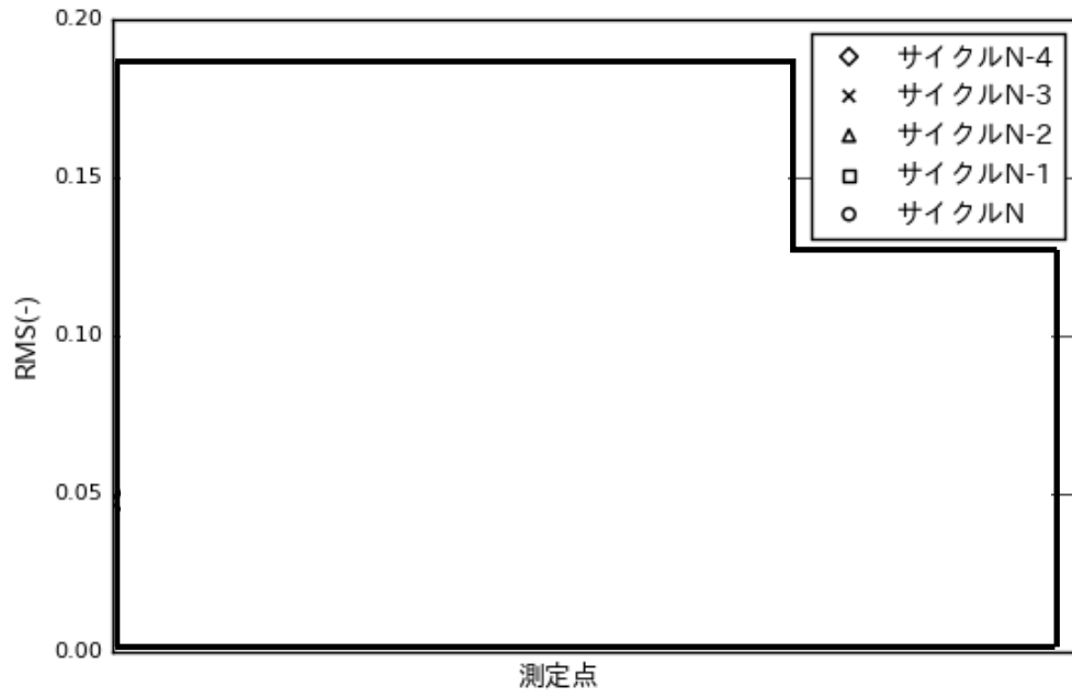
図 3-85 TIP 測定値と計算値の軸方向 RMS 差 (長期停止運転)
