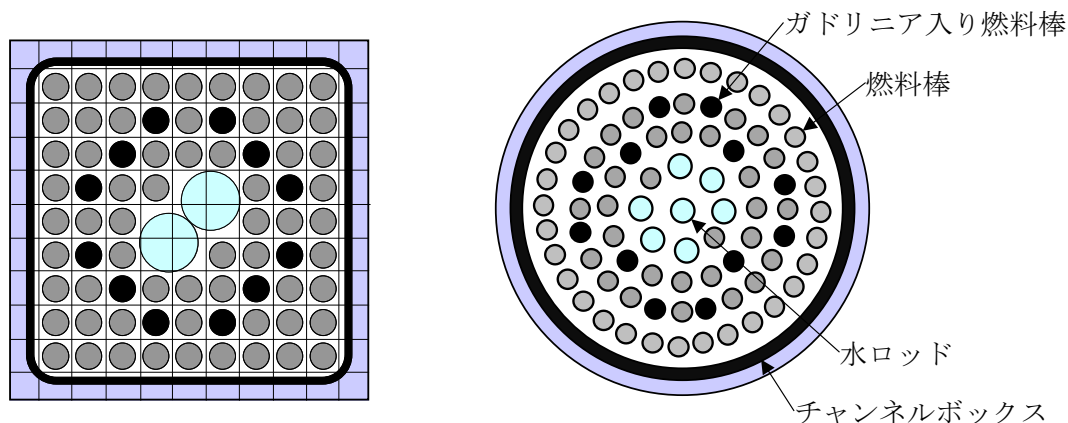
図 3.1-1 燃料集合体実形状と円筒クラスタ体系（ 9 \times 9 燃料の例）
