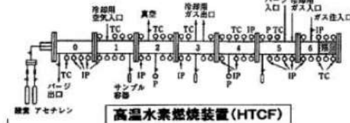
図2 NUPEC/U.S. NRC/BNL の高温燃焼試験 試験容器
