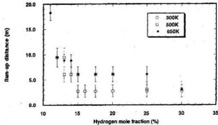
参考図3 NUPEC/U.S. NRC/BNL の高温燃焼試験で計測された助走距離
