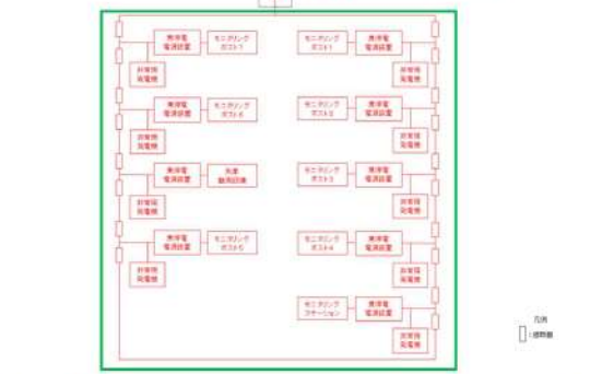
第1.1.2-1図 モニタリングポスト及びモニタリングステーションの電源構成概略図等 (1/2)
