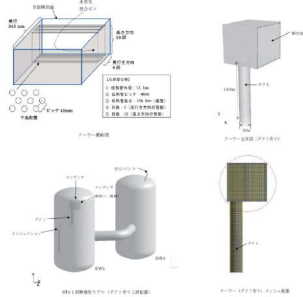
図1 PANDA試験の試験前解析モデル図
