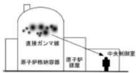
図7.6 原子炉冷却材喪失の直接ガンマ線の計算（PWR型原子炉施設）
