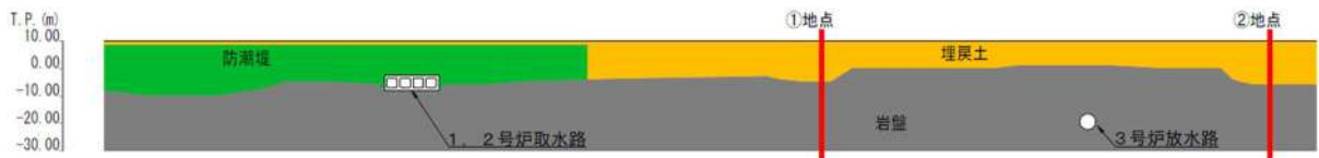
第 6-34 図 海岸付近 (A-A' エリア) の地質縦断図
