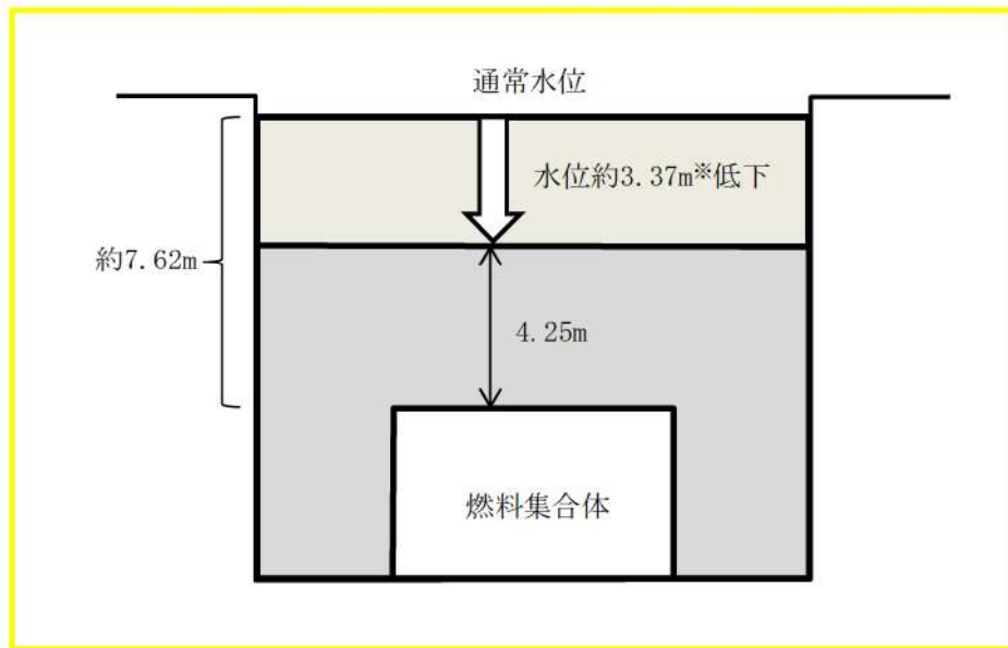
使用済燃料ピット水位概要図
