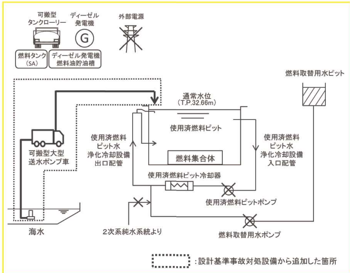
図1 想定事故1の重大事故等対策の概略系統図
