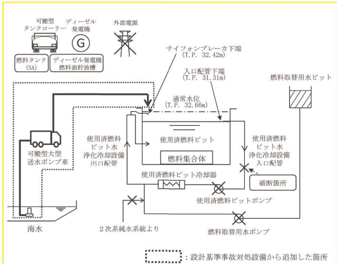
図1 想定事故2の重大事故等対策の概略系統図
