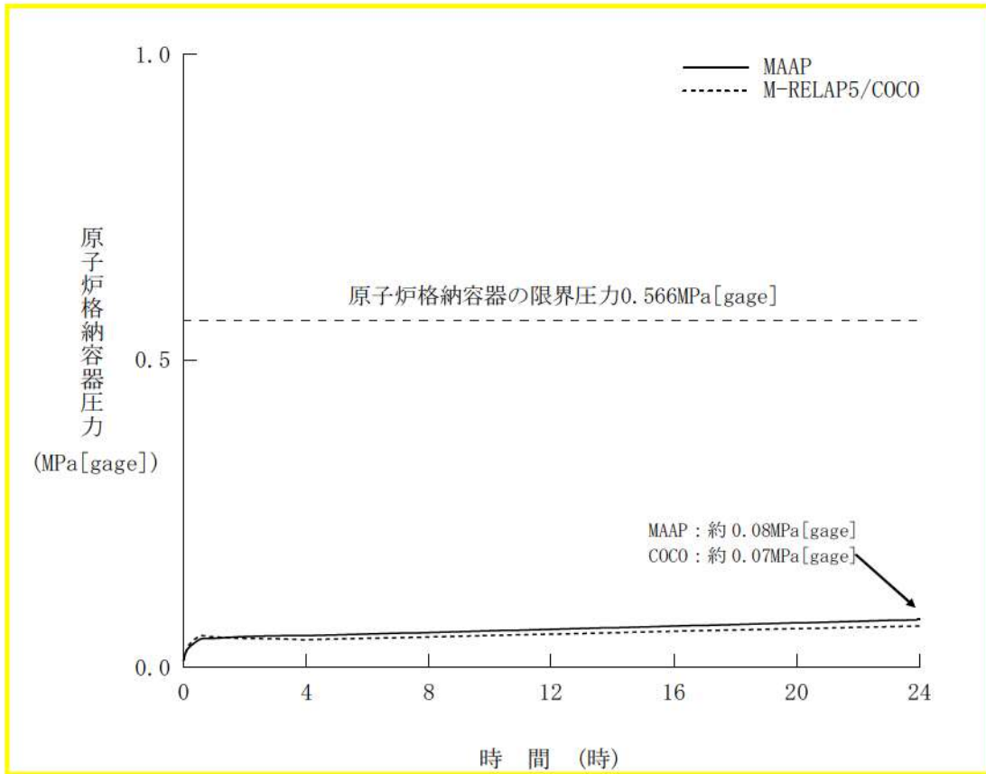
図5 原子炉格納容器圧力の推移比較(24時間)
