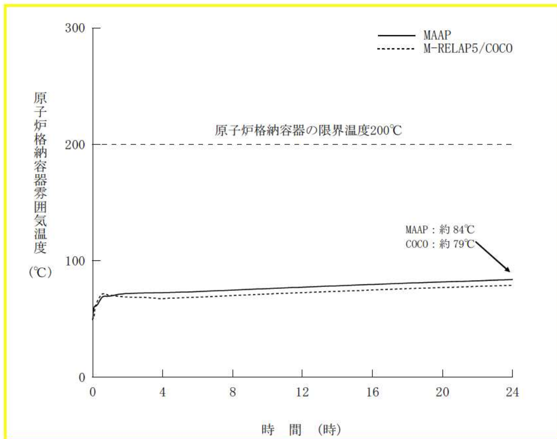
図6 原子炉格納容器雰囲気温度の推移比較(24時間)
