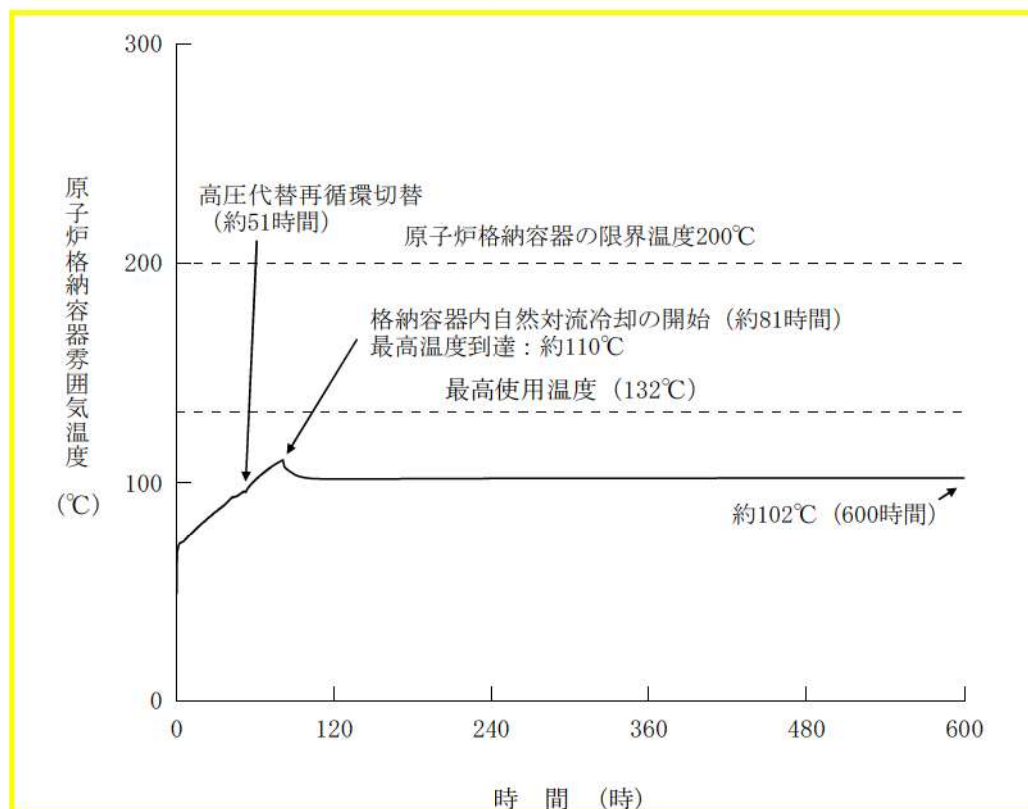
図4 原子炉格納容器雰囲気温度の推移 (確認解析2)
