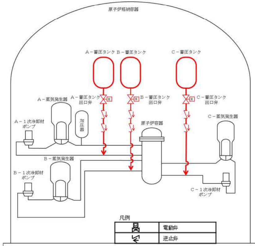
1次冷却系のフィードアンドブリード（蓄圧注入系による注水）
