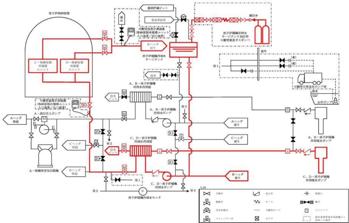
第40-1図 格納容器内自然対流冷却（原子炉補機冷却水）系統概要図
