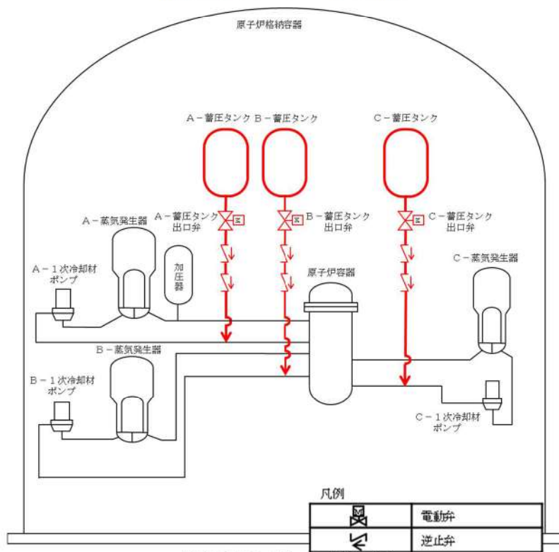
(蓄圧注入系による注水)
