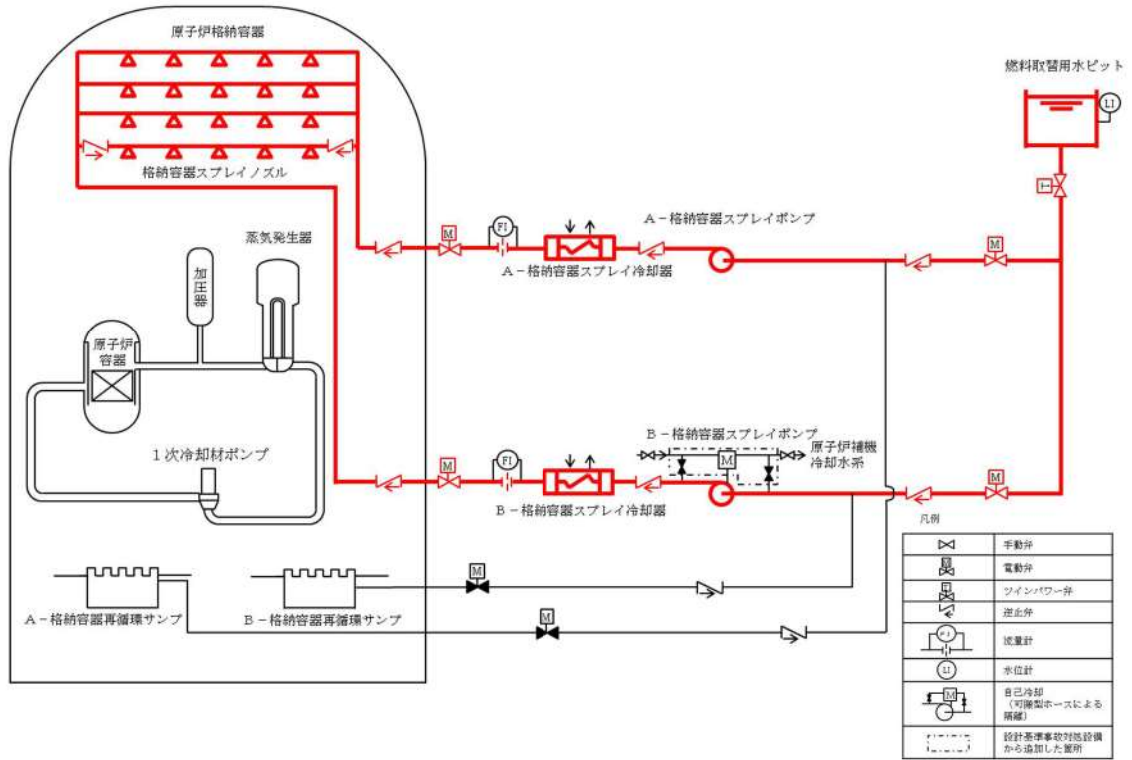
(格納容器スプレイ時)
