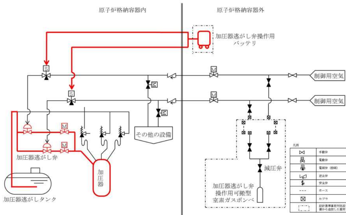
加圧器逃がし弁の機能回復
