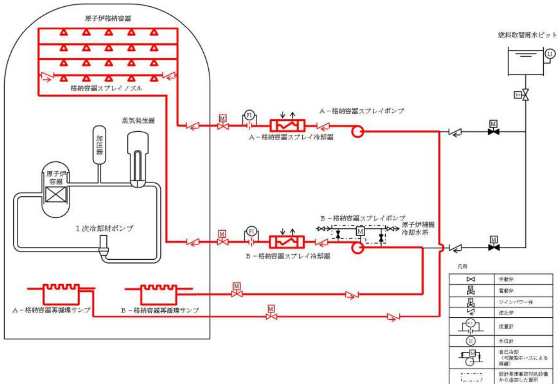
(格納容器再循環による格納容器スプレイ時)
