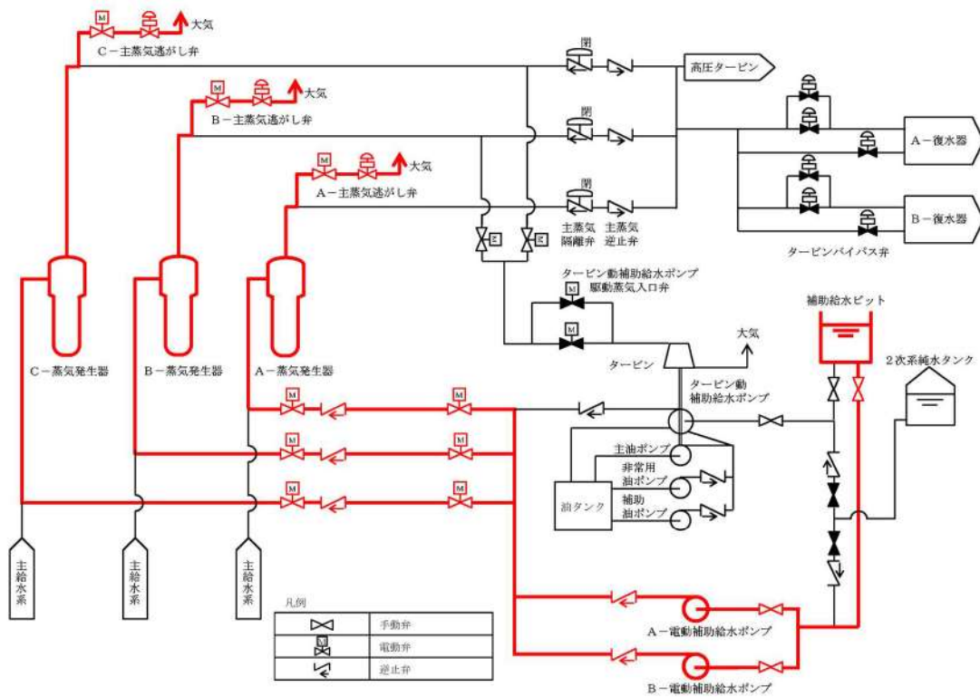
蒸気発生器 2 次側からの除熱（電動補助給水ポンプの機能回復）
