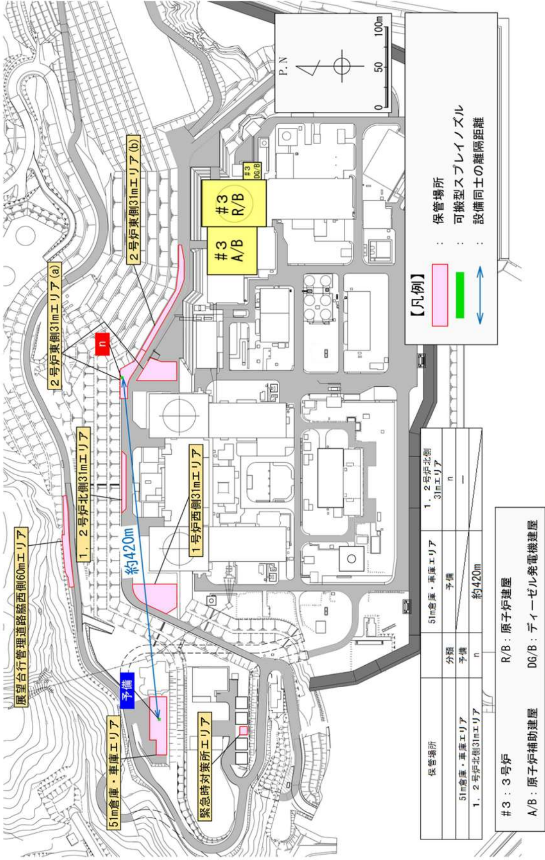
第 5-5 図 (2/2) 屋外重大事故等対処設備の位置的分散にかかるとる具体的な配置計画 (可搬型スプレインゾル : n)
