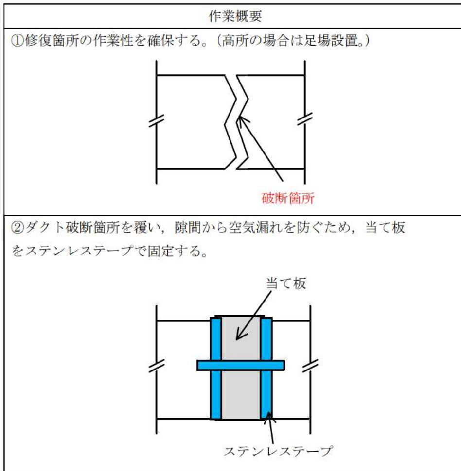
第2.1.2.4図 当て板による修復作業概要
