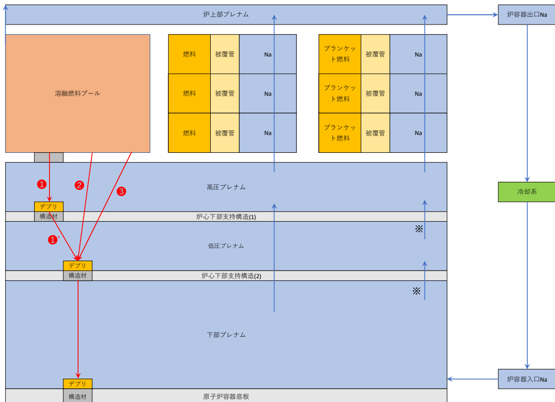
図1 ULOF による溶融燃料プール形成時の解析モデル概要
