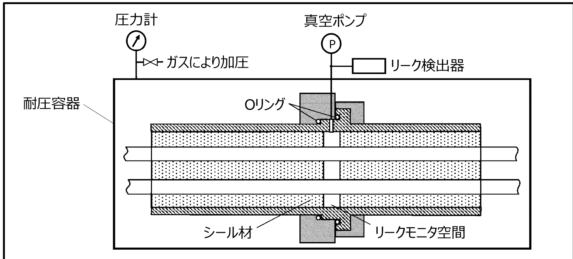
リーク量測定試験装置概略図
