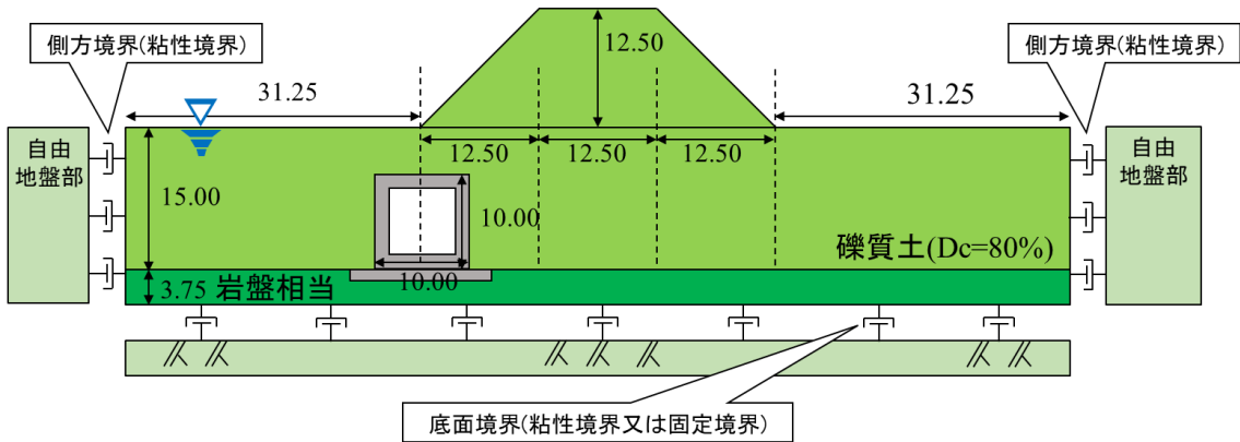
(解析モデル 2*：盛土・地中構造物有り)
