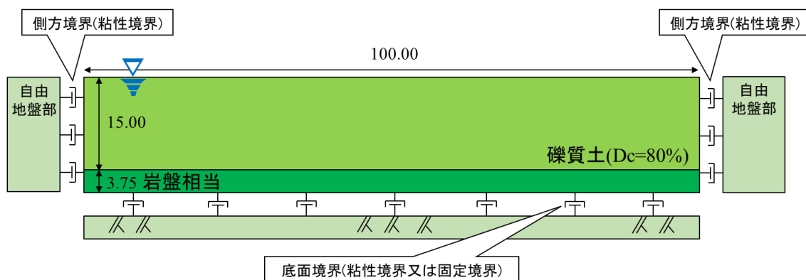
(解析モデル 3 : 成層地盤)
