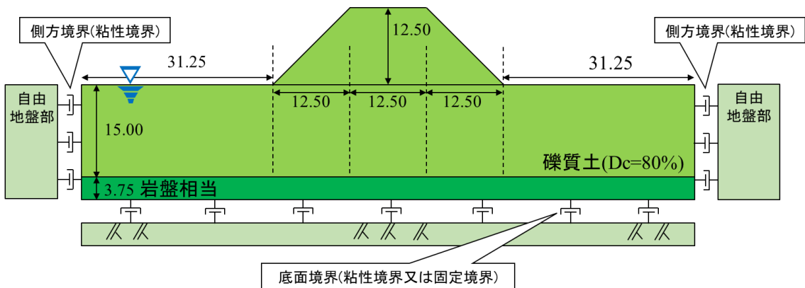
(解析モデル 1*：盛土有り・地中構造物なし)
