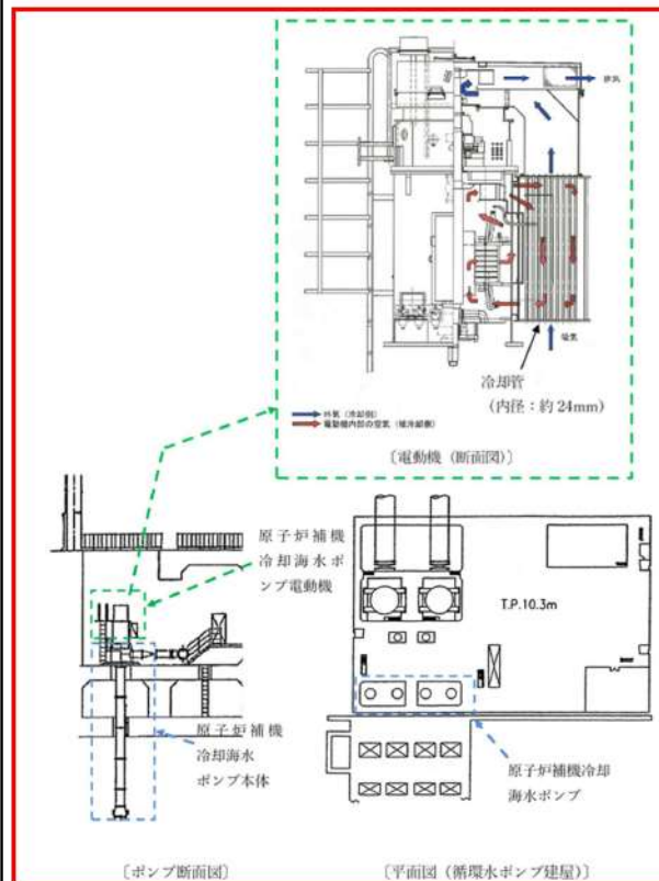
第8-1図 原子炉補機冷却海水ポンプ用電動機の冷却方式
