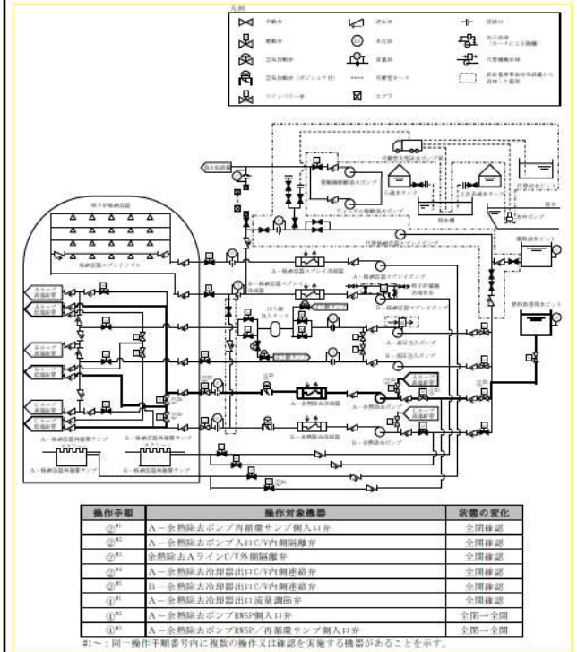
第1.4.39図 燃料取替用水ビットからの重力注水による原子炉容器への注水 概要図(2/2) (サポート系故障時)
