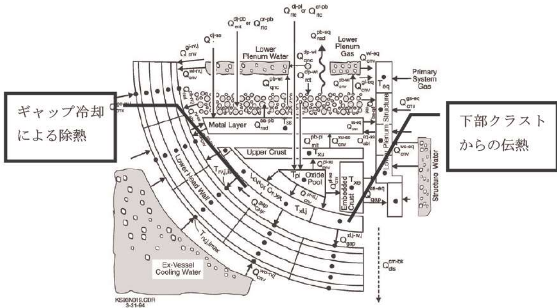
付図 4-1 下部プレナムでのエネルギー移行モデル 出典：MAAP4 User's Manual, EPRI
