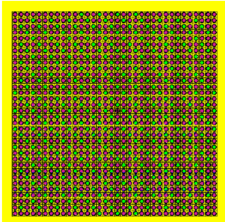
図1 燃料棒：コンクリート棒：SUS棒：水領域比率 800:0:356:0 (34×34)の炉心構成例
