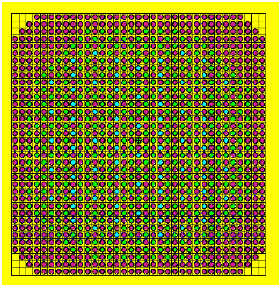
図 2 燃料棒：コンクリート棒：SUS 棒：水領域比率 800:80:356:24(36×35)の炉心構成例
