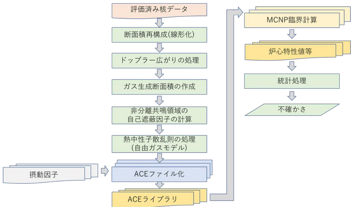
図3 ランダムサンプリング法による不確かさ評価の流れ
