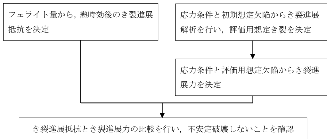
図 2 熱時効評価の流れ
