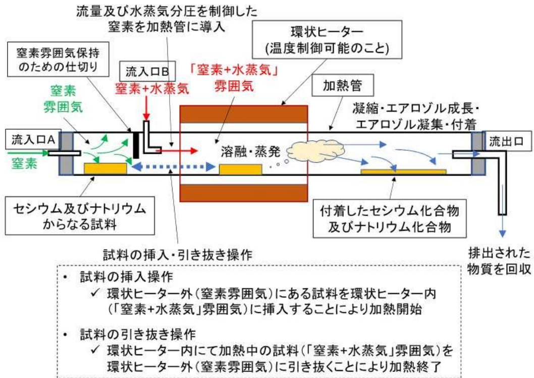
図 1: アルカリ金属蒸発試験装置の概念図
