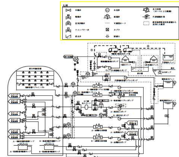
第1.8-12図 代替循環冷却系による原子炉格納容器下部への注水 概要図 (1/2)
