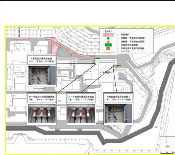
第3図 建屋接続場所(3/8)
