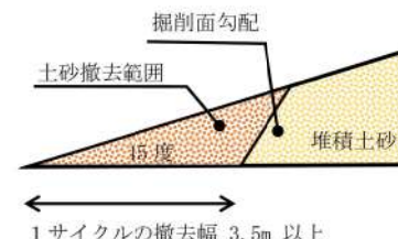
第6図 掘削面のイメージ
