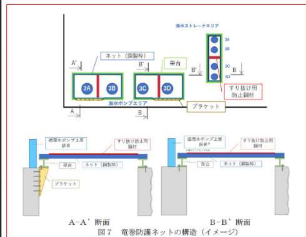
図7 竜巻防護ネットの構造（イメージ）
