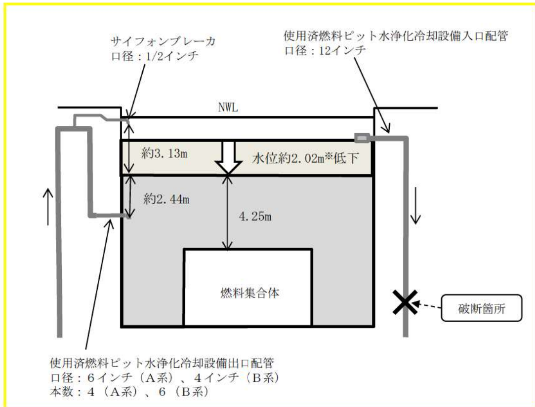
使用済燃料ピット水位概要図
