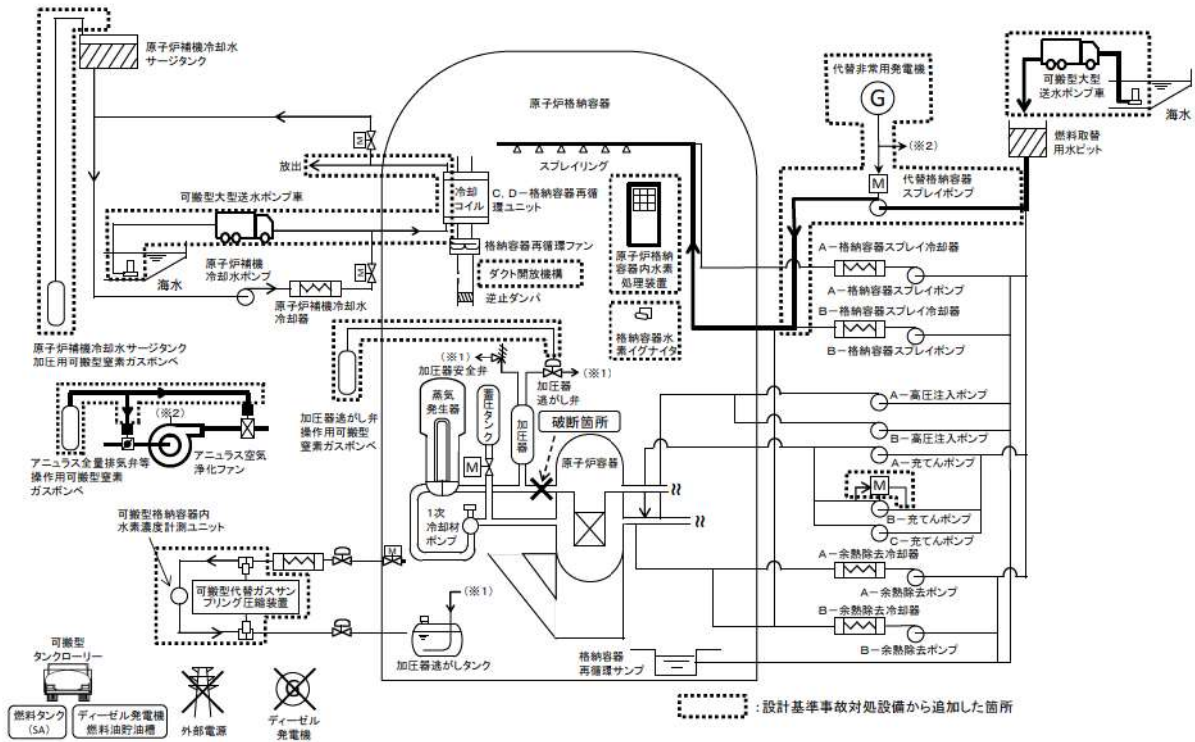
第 7.2.1.1.1 図 「雰囲気圧力・温度による静的負荷（格納容器過圧破損）」 の重大事故等対策の概略系統図（1 / 2）（代替格納容器スプレィ）
