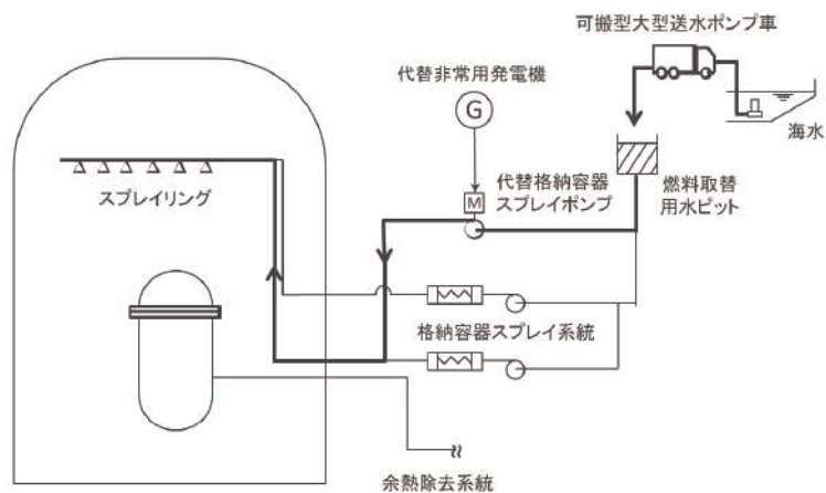
図 1 概略系統図
