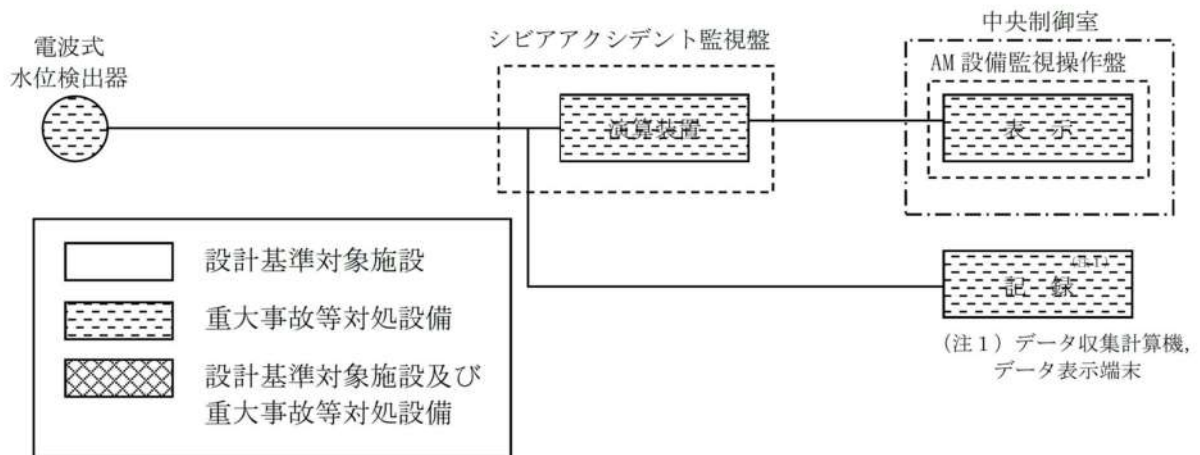
第 37 図 使用済燃料ピット水位 (AM 用) の概略構成図
