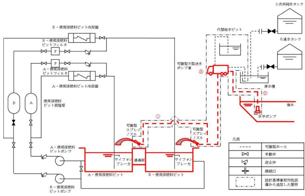
図 54-4-2 使用済燃料ピットへのスプレイ
