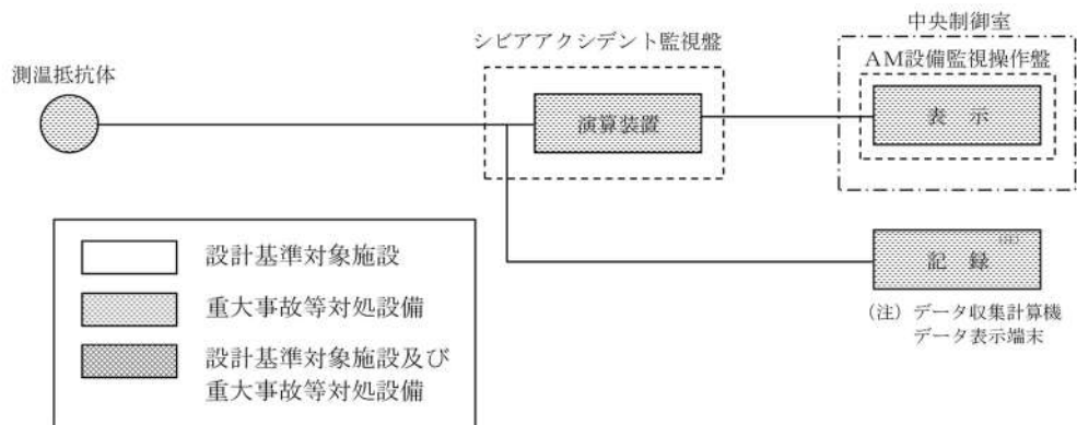
第3図 使用済燃料ピット温度（AM用）の概略構成図
