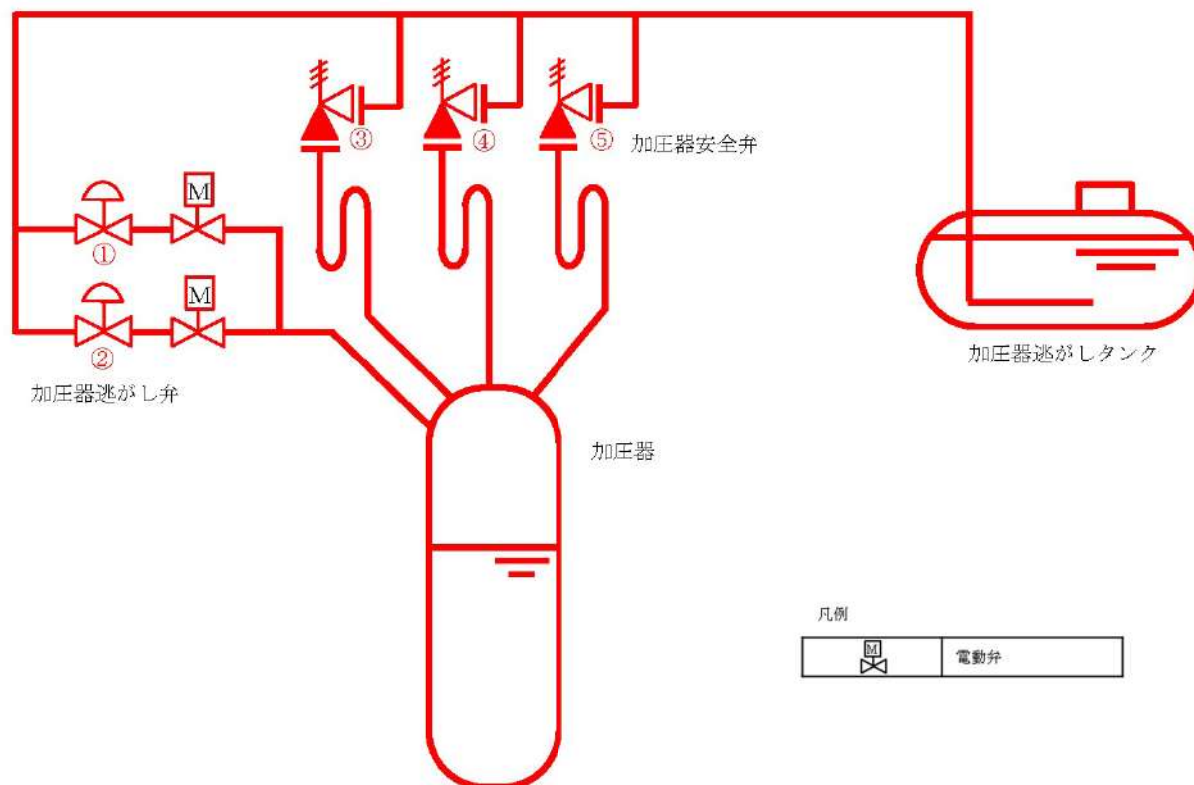
図 44-4-4 原子炉出力抑制 (3)
