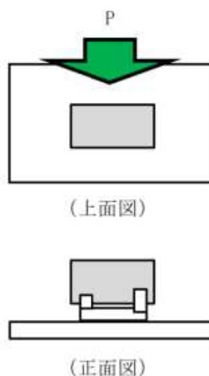
別添 1 - 2 - 1 図 津波荷重の作用方向（径方向衝突の場合）
