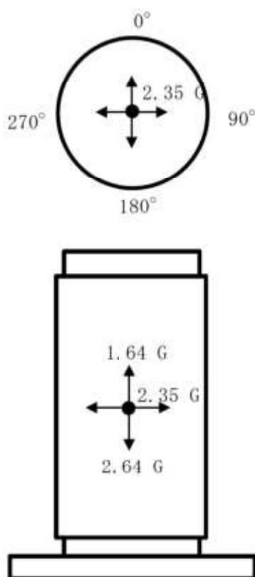
別添 2-2-7 図 地震力の作用方向 (基礎等に固定する設置方法)
