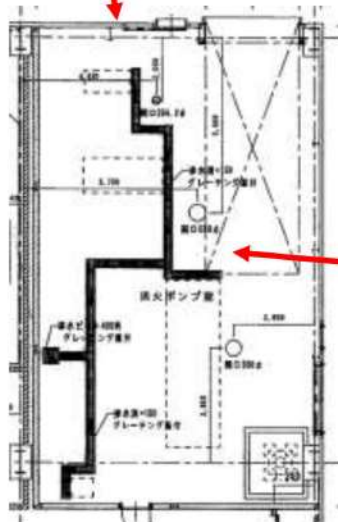
第 1-23 図：消火ポンプ設置エリアの風水害対策
