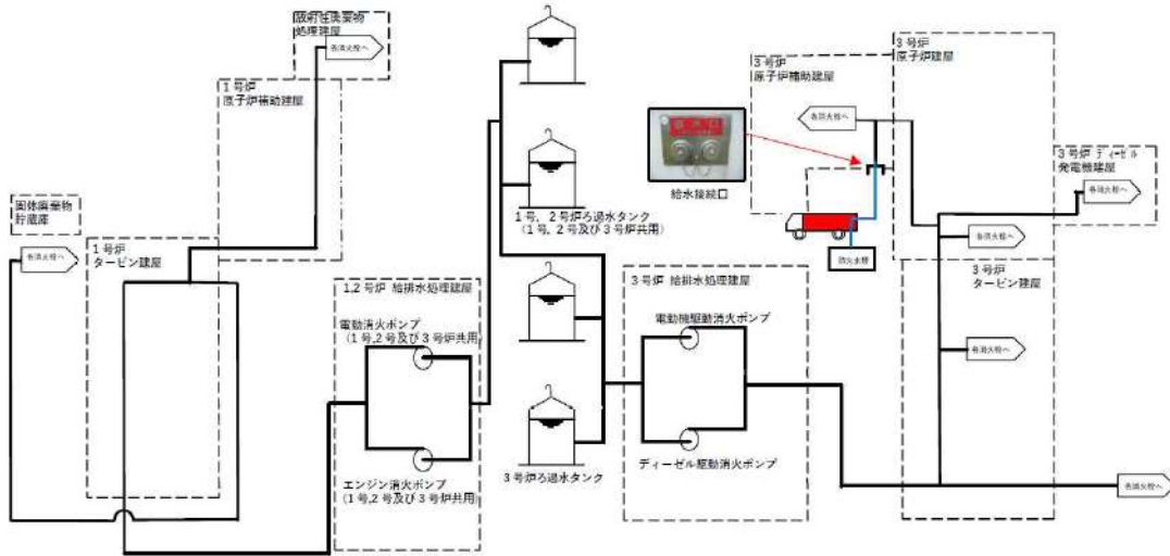
第 1-24 図：給水接続口接続概要図
