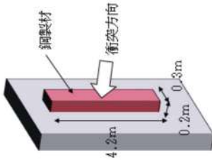
第3.3.1.2図 最大衝撃荷重となる鋼製材衝突方向 (Rieraの方法 (1) )
