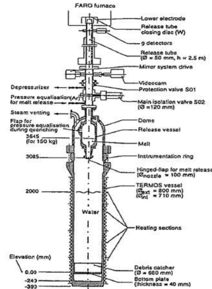
図3.1-1 FARO 実験装置
