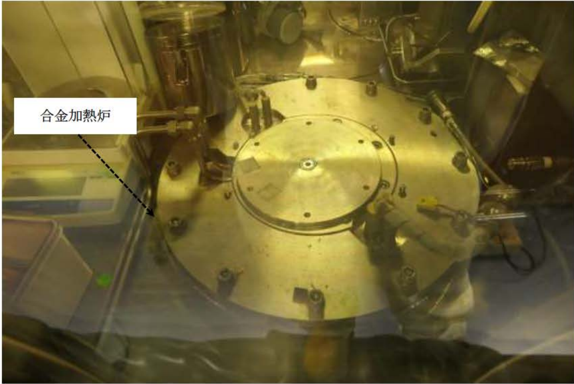
図-2-12 合金加熱炉 (124-D グローブボックス) の外観
