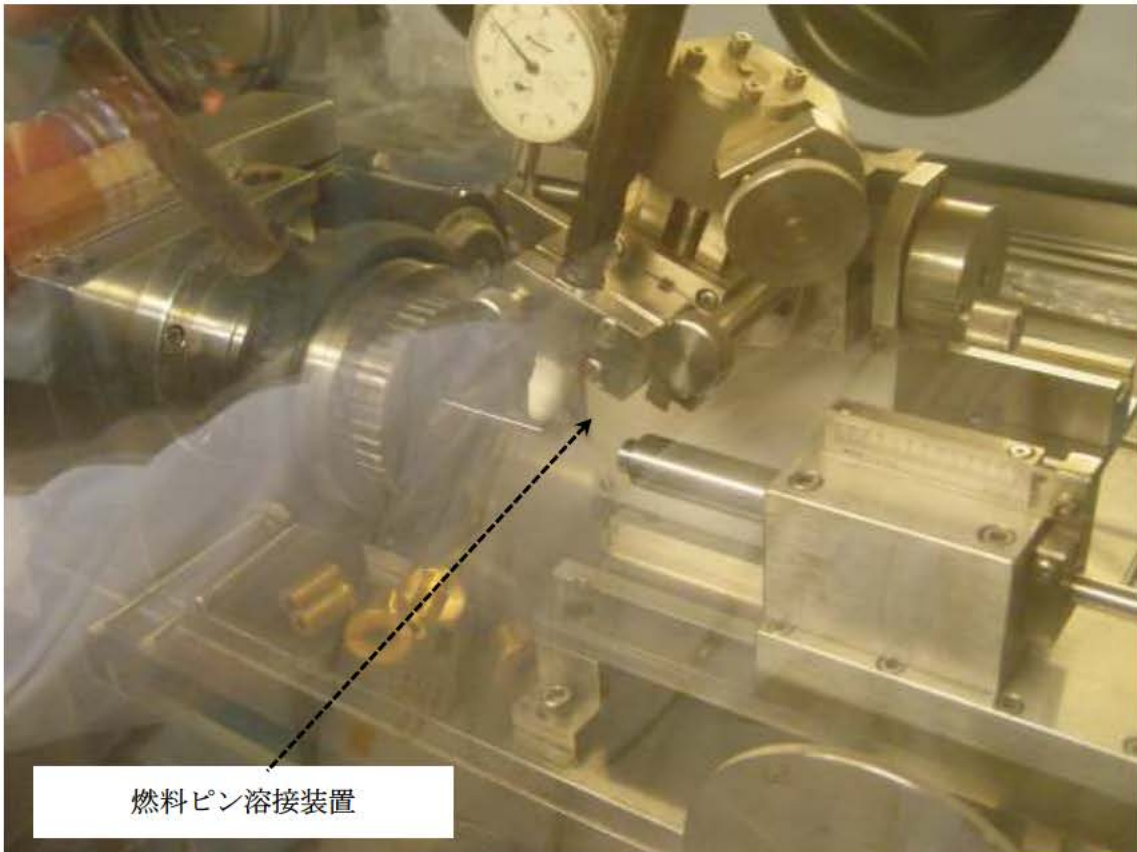
図-2-26 燃料ピン溶接装置 (902-D グローブボックス) の外観
