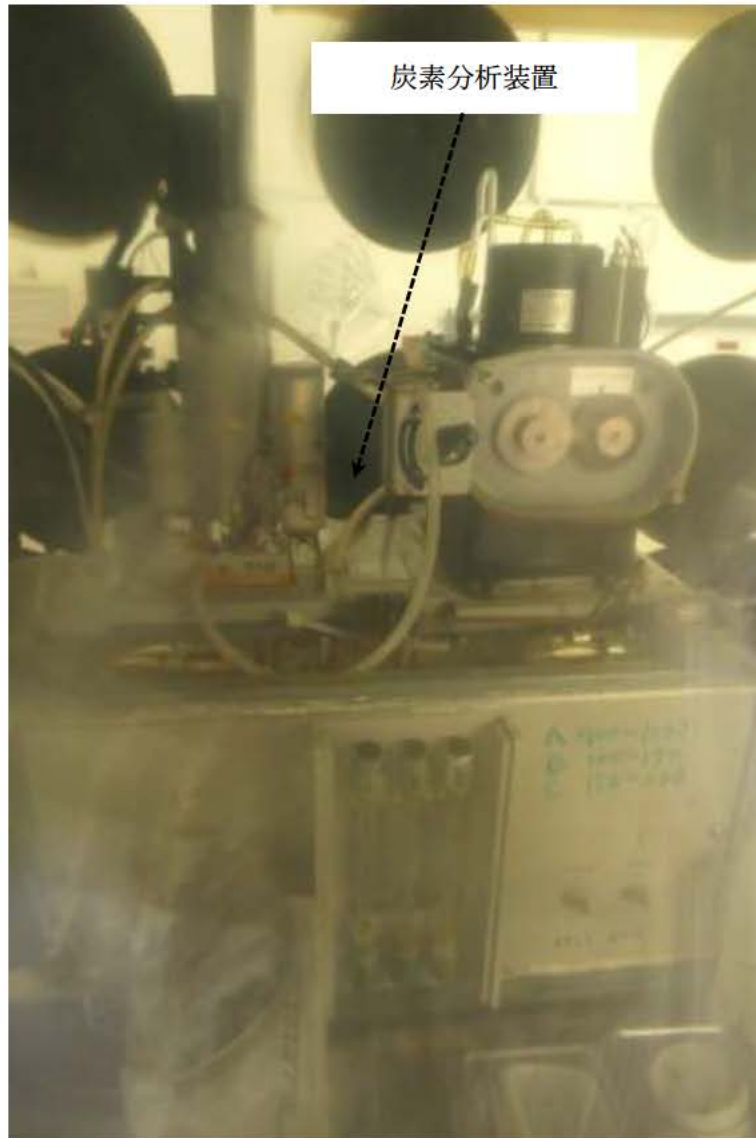
図-2-25 炭素分析装置 (821-D グローブボックス) の外観
