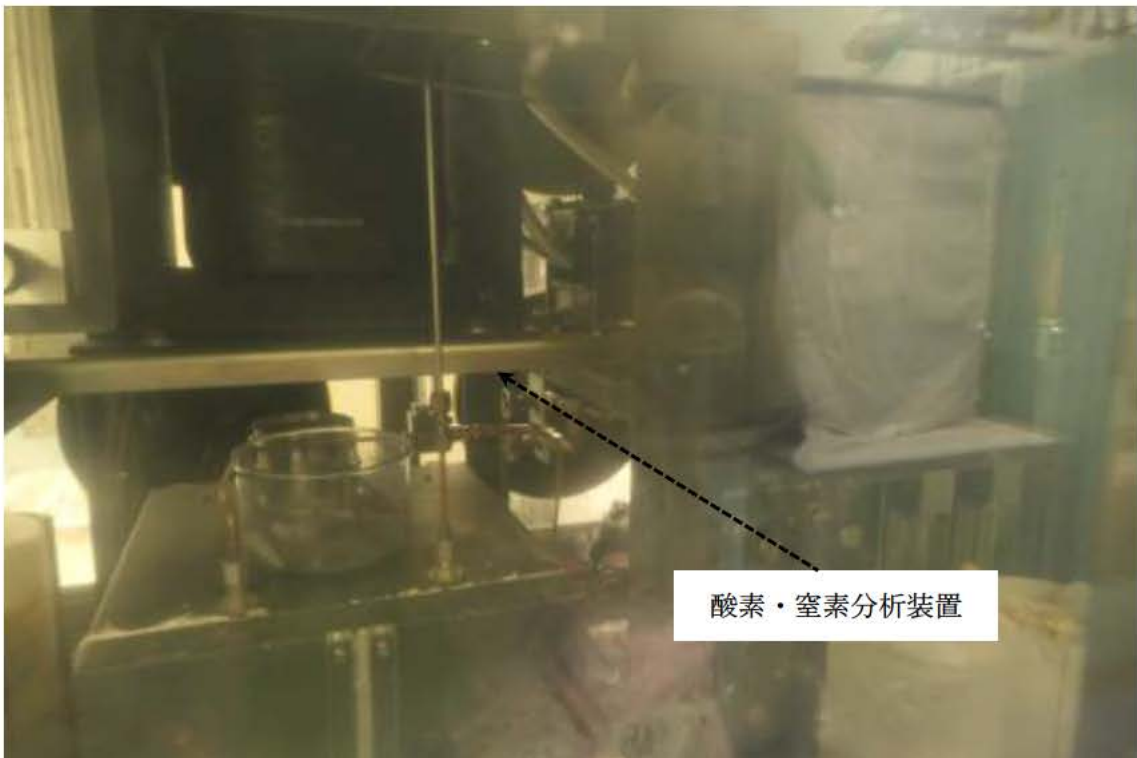
図-2-24 酸素・窒素分析装置 (811-D グローブボックス) の外観
