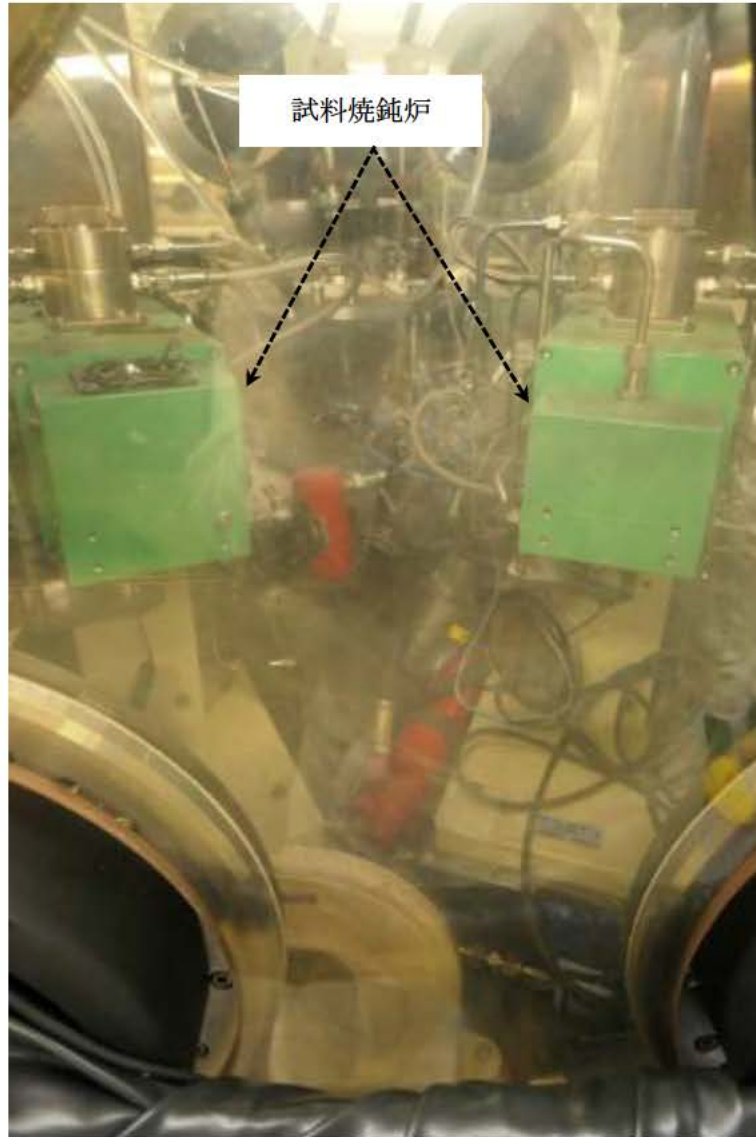
図-2-9 試料焼鈍炉（115-D グローブボックス）の外観
