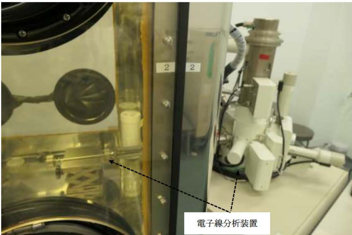
図-2-22 電子線分析装置 (702-D グローブボックス) の外観
