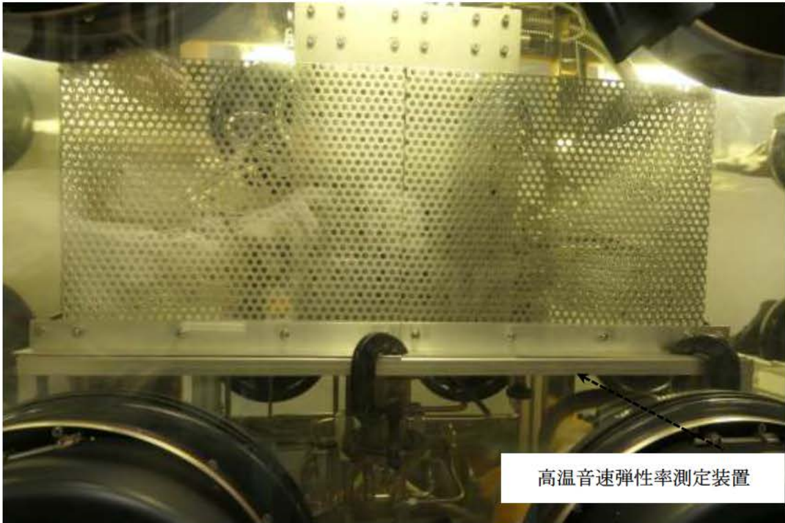
図-2-23 高温音速弾性率測定装置 (711-D グローブボックス) の外観
