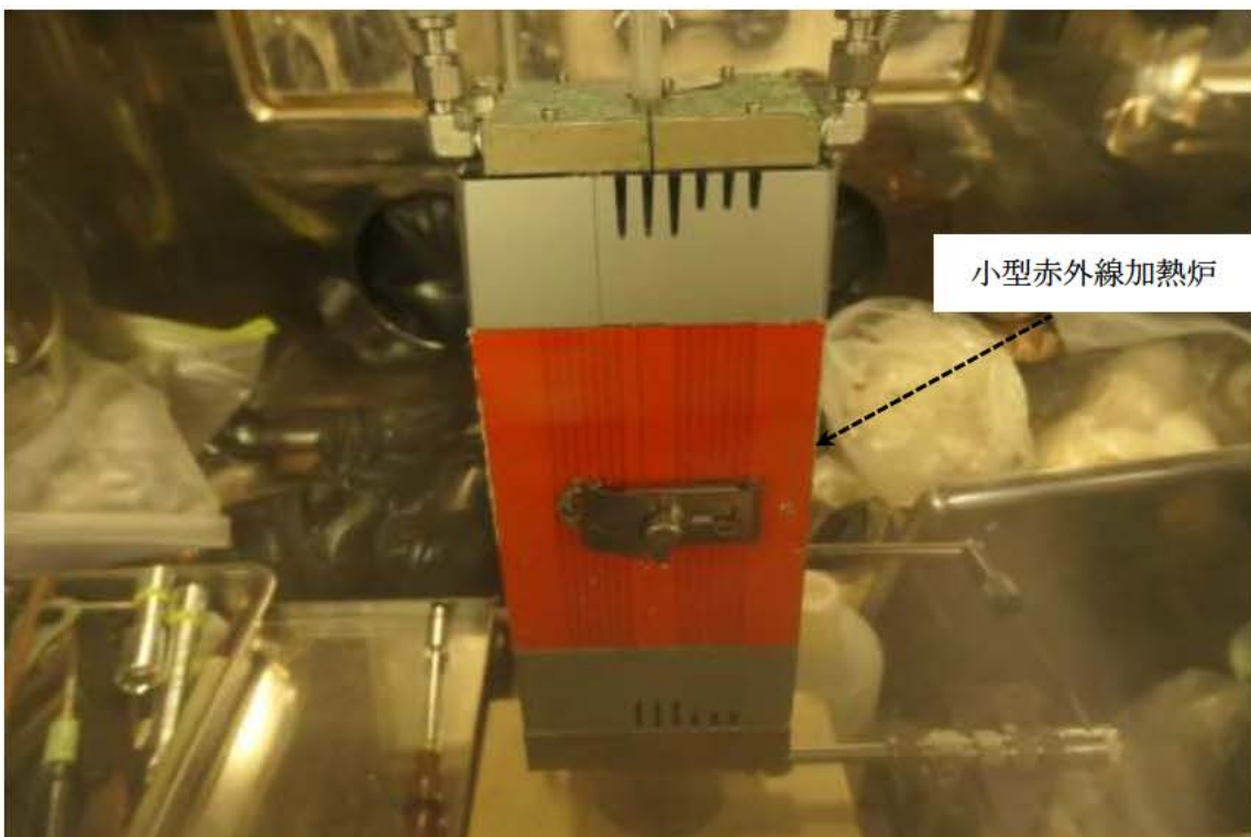
図-2-2 小型赤外線加熱炉 (102-D グローブボックス) の外観
