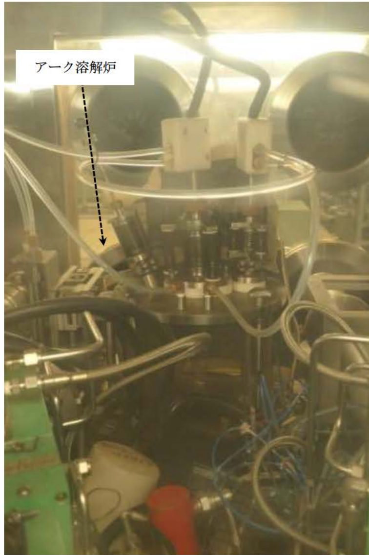
図-2-8 アーク溶解炉（115-D グローブボックス）の外観
