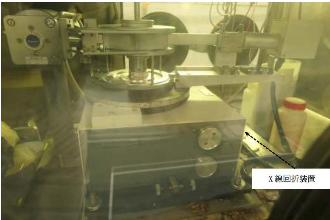
図-2-19 X線回折装置 (302-D グローブボックス) の外観
