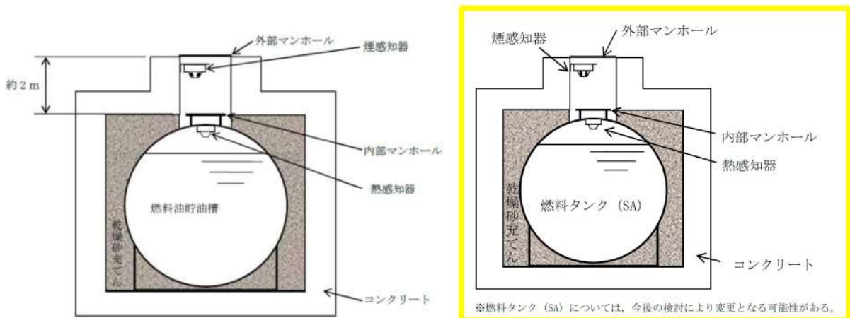
第 41-4-1 図 ディーゼル発電機燃料油貯油槽及び燃料タンク (SA) の火災感知器設置概要図
