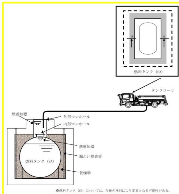
第3図：燃料タンク (SA) の構造及び給油イメージ (A-A' 矢視)
