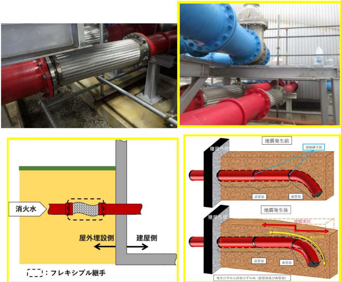
第 41-1-25 図 地盤変位対策の実施例
