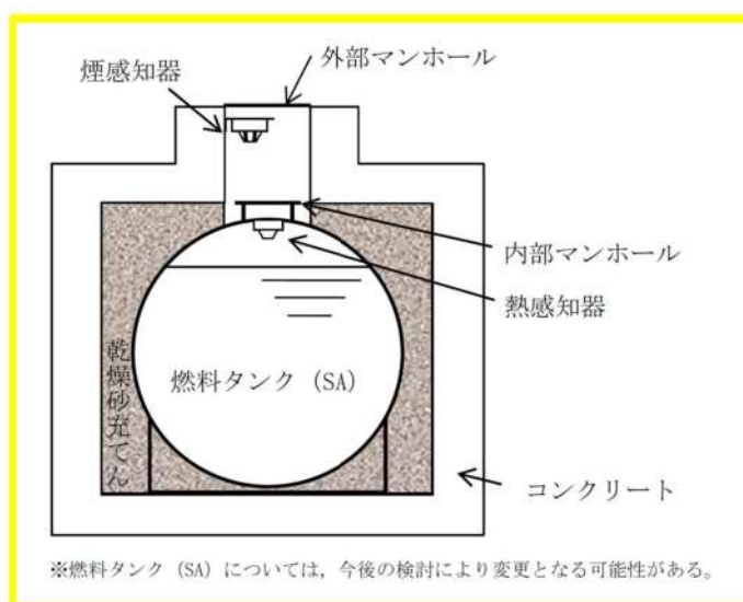
第 41-1-12 図：火災感知器設置概要
