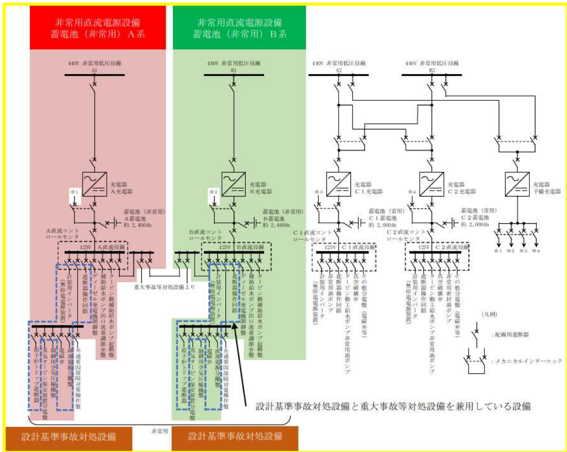
第 4 図 直流電源設備の遮断器とメカニカルインターロックによる分離
