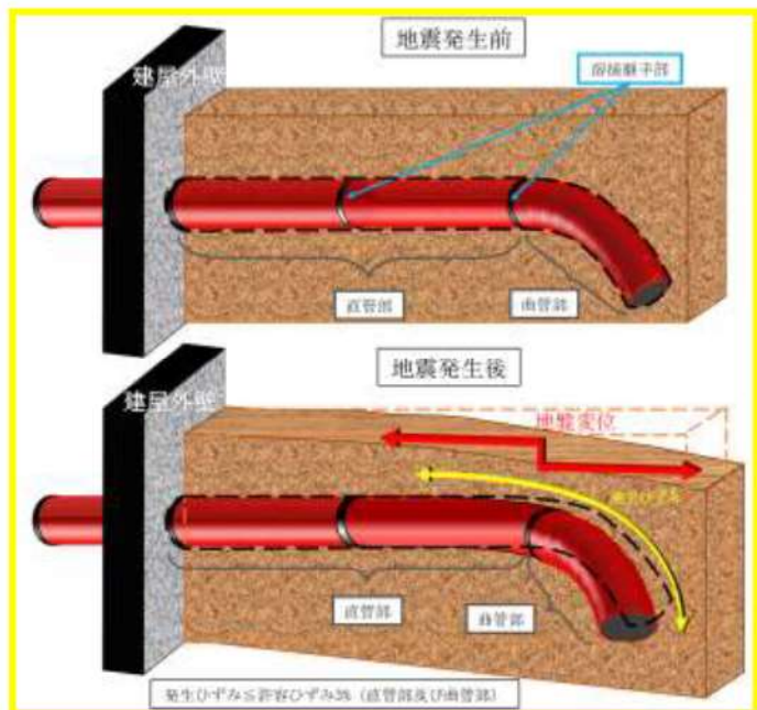
第 1-23 図：地震変位対策の実施例
