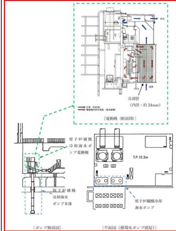
図8-1 原子炉補機冷却海水ポンプ用電動機の冷却方式
