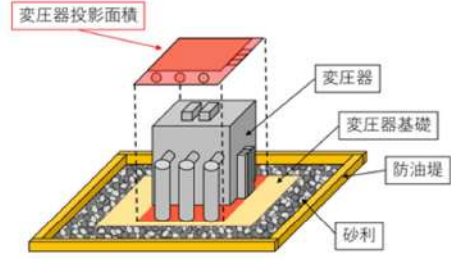
図6-10 変圧器の投影面積
